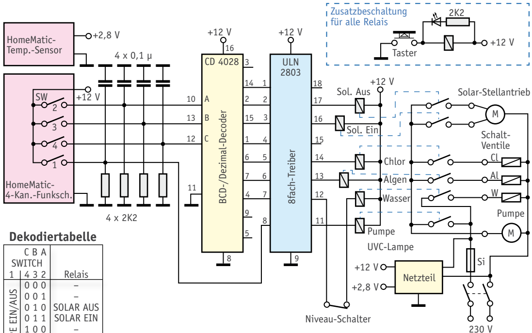
Bild 4: Der Schaltplan der Steuerung, links die Dekodiertabelle für die Schalterfunktionen
