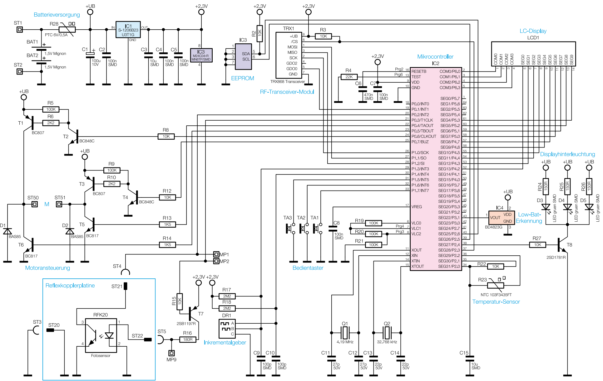
Bild 2: Schaltbild des MAX: Heizkörperthermostaten
