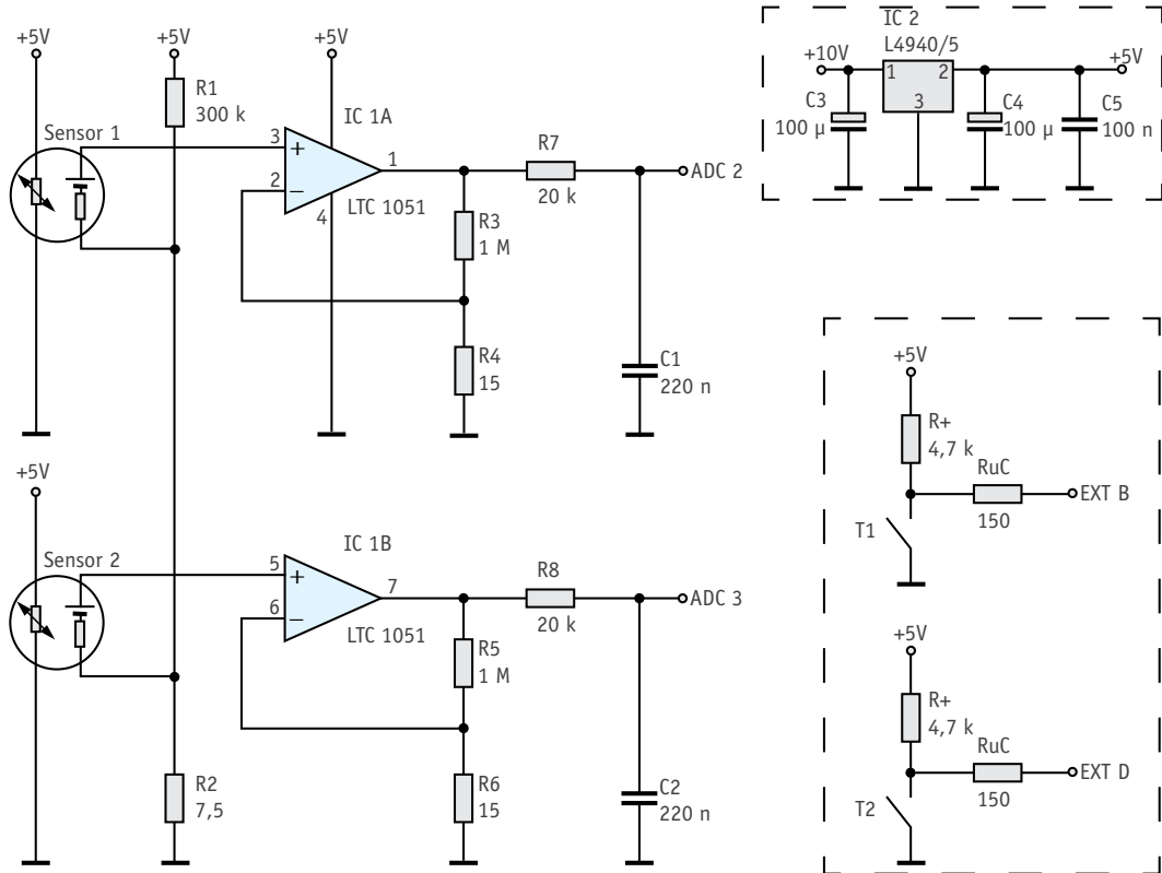
Bild 2: Die Gesamtschaltung der Zusatzplatine
