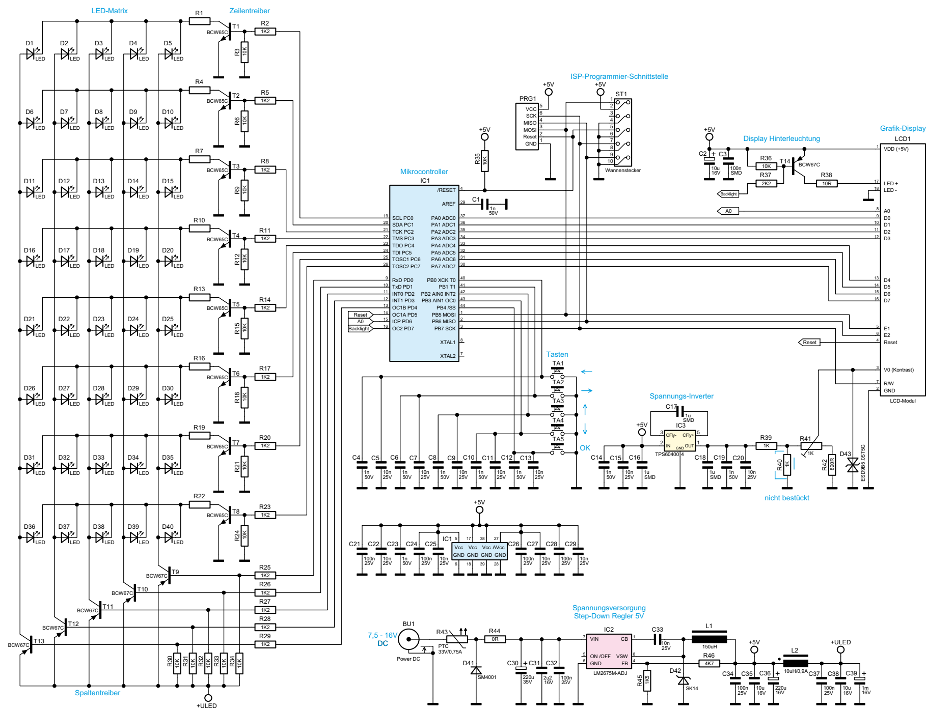
Bild 3: Die Gesamtschaltung des LBH40. Die Vorwiderstände der LEDs sind entsprechend der Beschreibung im Text zu dimensionieren.
