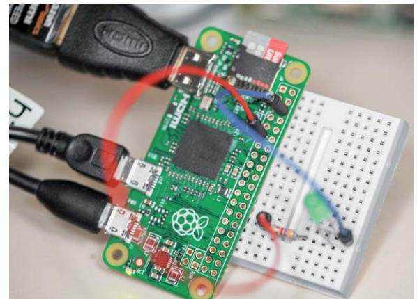
Bild 1: Für kleine Schaltungsexperimente kann der Raspberry Pi Zero auch mal direkt an das Breadboard gesteckt werden.
