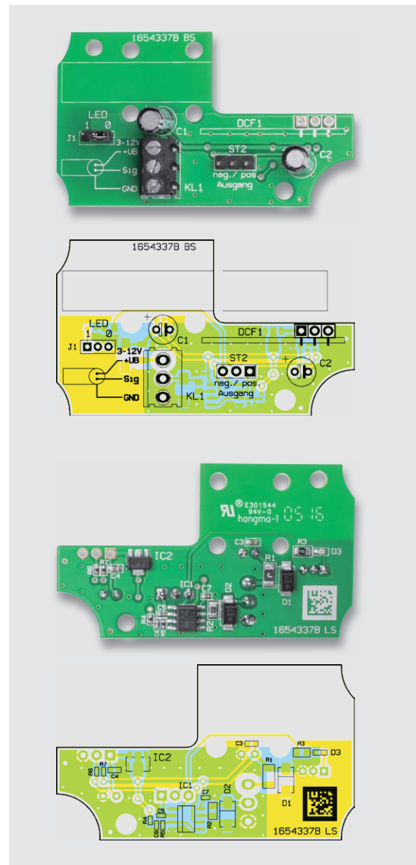
Bild 5: Die Platinenfotos und die Bestückungspläne des DCF-Moduls; oben die Oberseite mit bedrahteten Bauteilen, unten die Unterseite mit SMD-Bestückung
