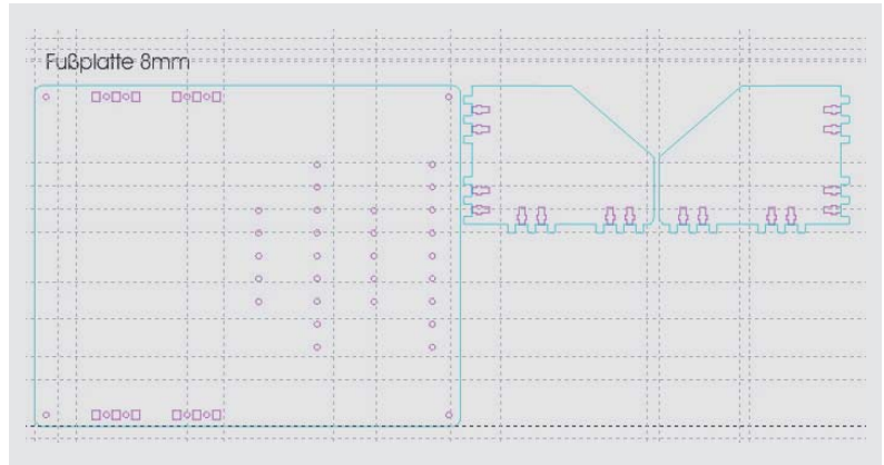
Bild 2: So sieht die Konstruktionszeichnung für die Fußplatte aus.
