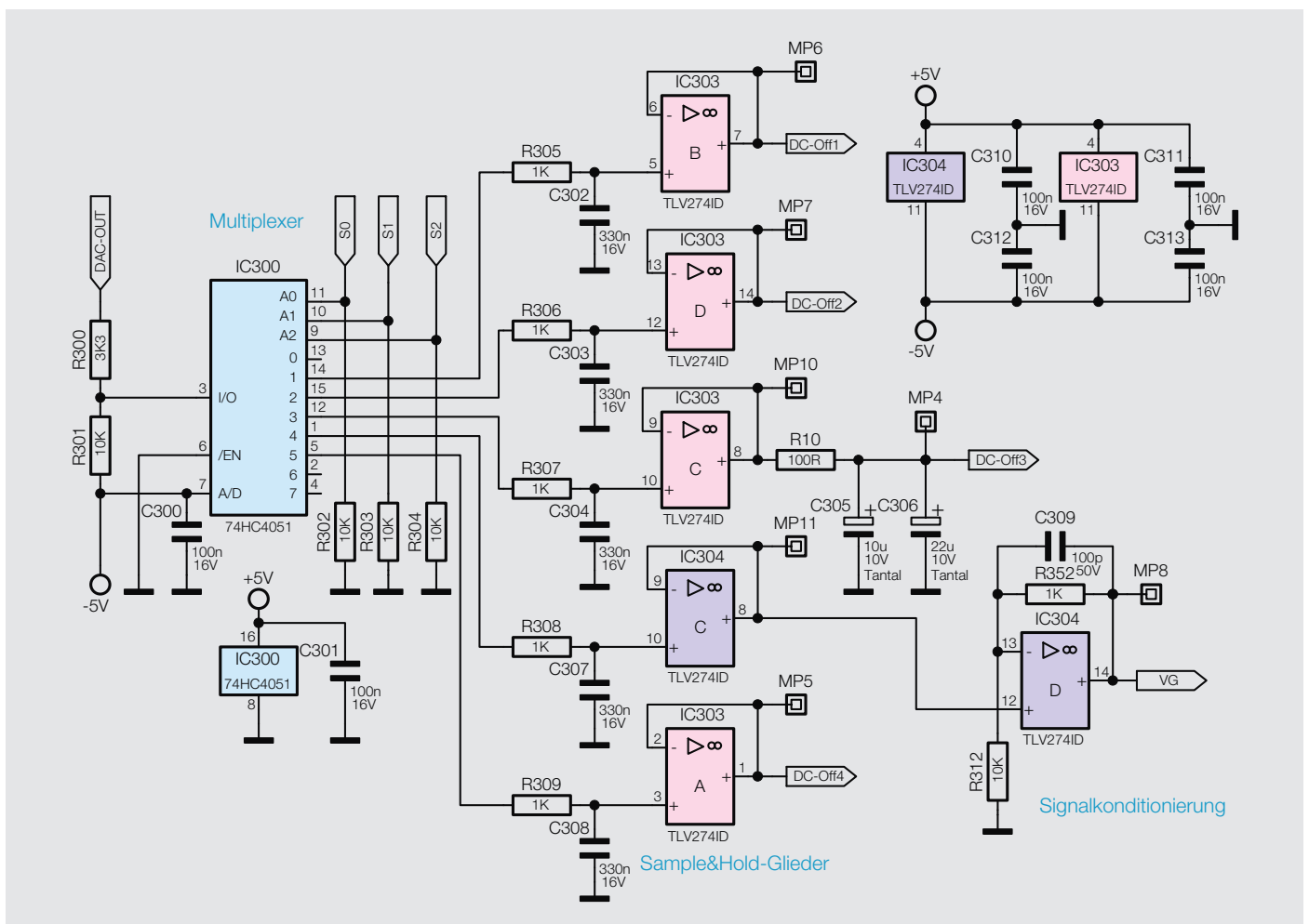
Bild 6: Die Sample-and-Hold-Schaltung
