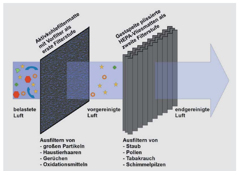
Bild 6: Die Hintereinanderschaltung eines Aktivkohlefilters und eines HEPA-Filters beseitigt bis zu 99,98 % der Luftschadstoffe mit weniger als 0,3 µm Durchmesser.
