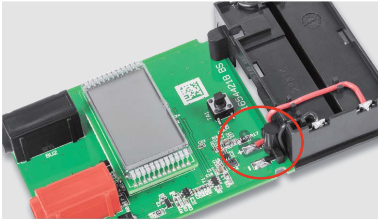
Bild 16: Die Anschlussdrhte des Batteriehalters werden, wie hier gezeigt, mit den Ltspads ST2 (rot, +) und ST3 (schwarz, -) verltet.
