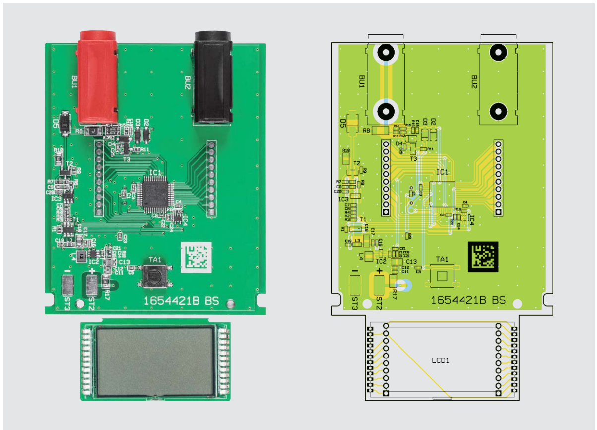
Bild 2: Platinenfoto der Haupt- und Displayplatine des BT100 mit zugehörigem Bestückungsplan
