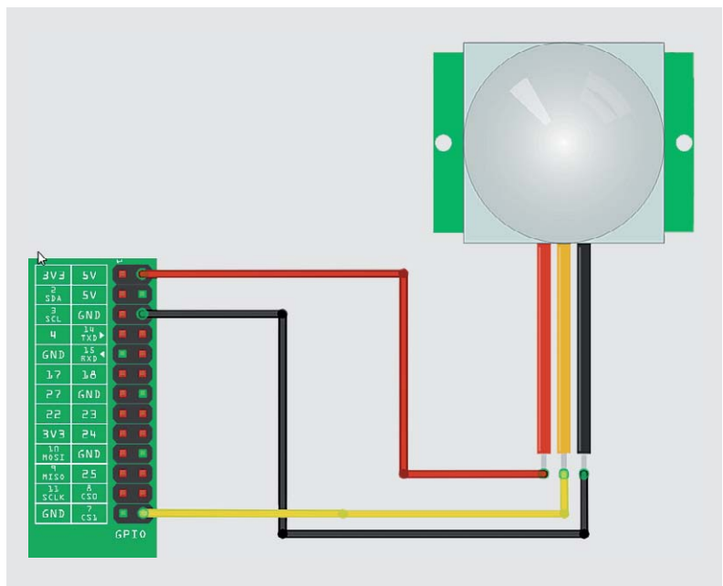
Bild 14: Neben Spannung und Masse benötigt der PIR-Sensor einen Dateneingang auf der GPIO-Leiste – hier wird GPIO7 genutzt.
