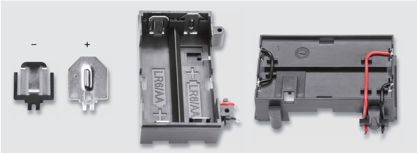
Bild 15: Die Batteriekontakte sind, wie hier gezeigt, in den Batterierhalter einzusetzen und zu verdrahten.
