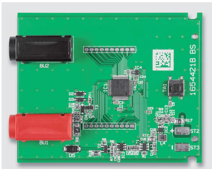
Bild 10: So erfolgt die richtige Bestückung der Messbuchsen.
