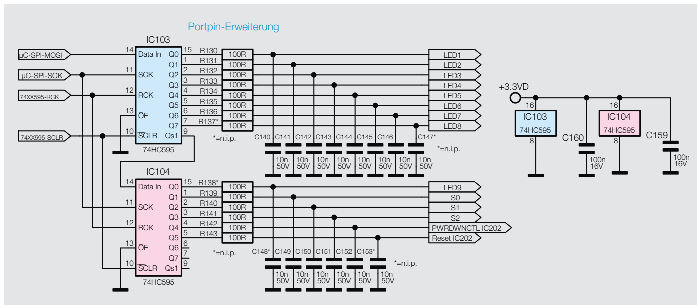
Bild 5: Schaltbild der beim DDS 8100 eingesetzten Portpin-Erweiterung
