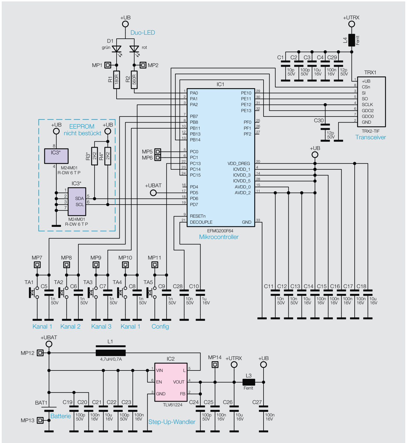
Bild 1: Das Schaltbild des Homematic Funk-Handsenders
