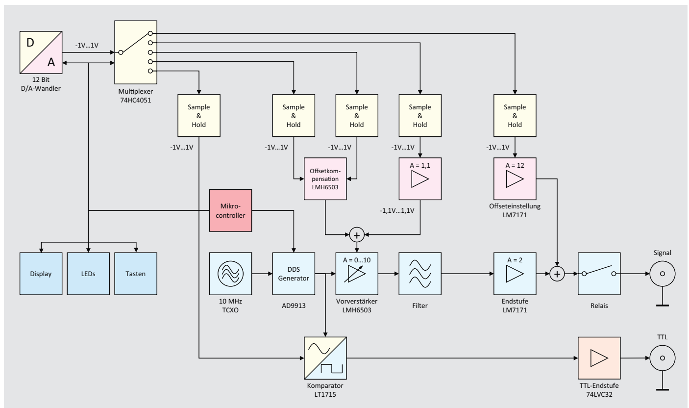
Bild 1: Blockschaftbild des DDS 8100
