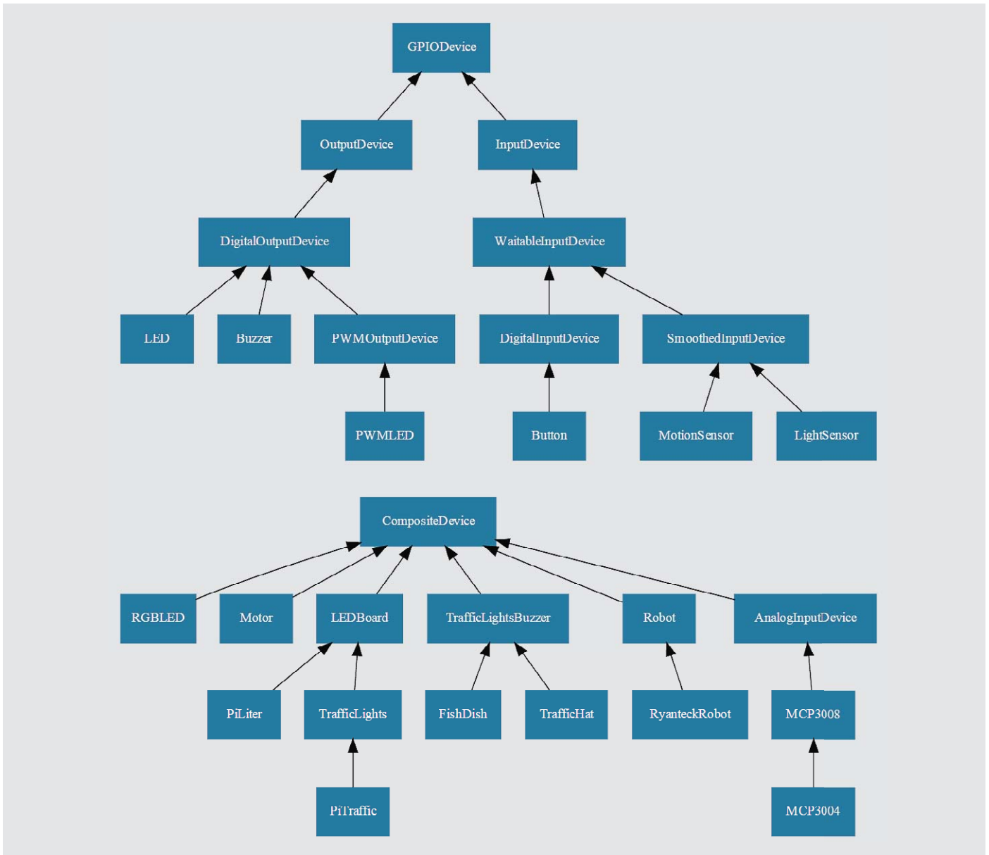
Bild 17: Dokumentation der gpiozero-Bibliothek ( https://gpiozero.readthedocs.org/en/rest-docs/api_generic.html ): Neben den in den Beispielen verwendeten LED- und MotionSensor-Klassen sind noch zahlreiche weitere Klassen in der API definiert.
