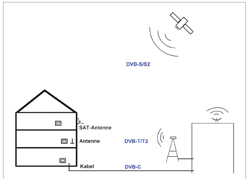
Bild 1: TV-Empfangswege
