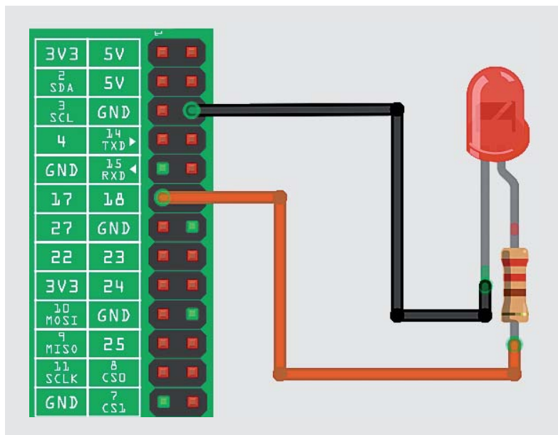
Bild 6: Die Schaltung für die LED ist auf dem Steckboard schnell umgesetzt.
