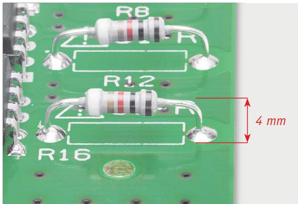
Bild 5: Die Widerstände R4, R8, R12 und R16 müssen in einem Abstand von 4 mm zur Platine montiert werden.
