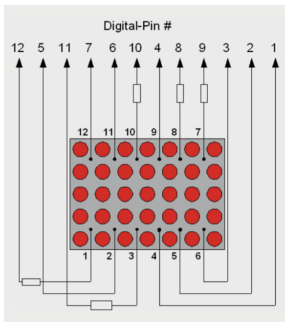
Bild 4: Schaltbild zum Anschluss der LED-Matrix an den Arduino
