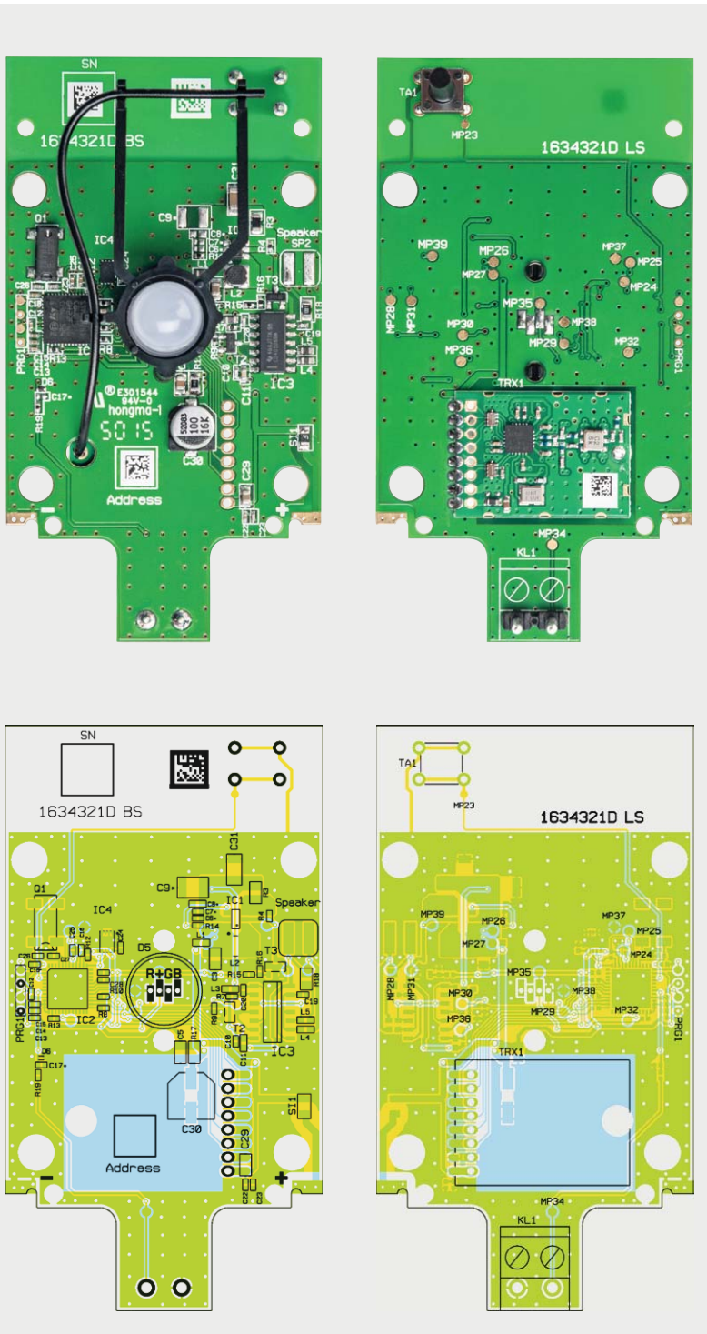
Bild 5: Platinfotos und Bestückungszeichnungen der Hauptplatine. Zur Lage der Antenne siehe Text.
