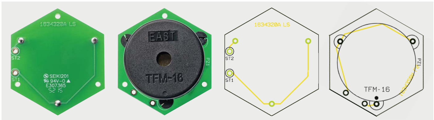
Bild 4: Platinfoto und Bestückungszeichnung der Piezo-Signalgeber-Platine
