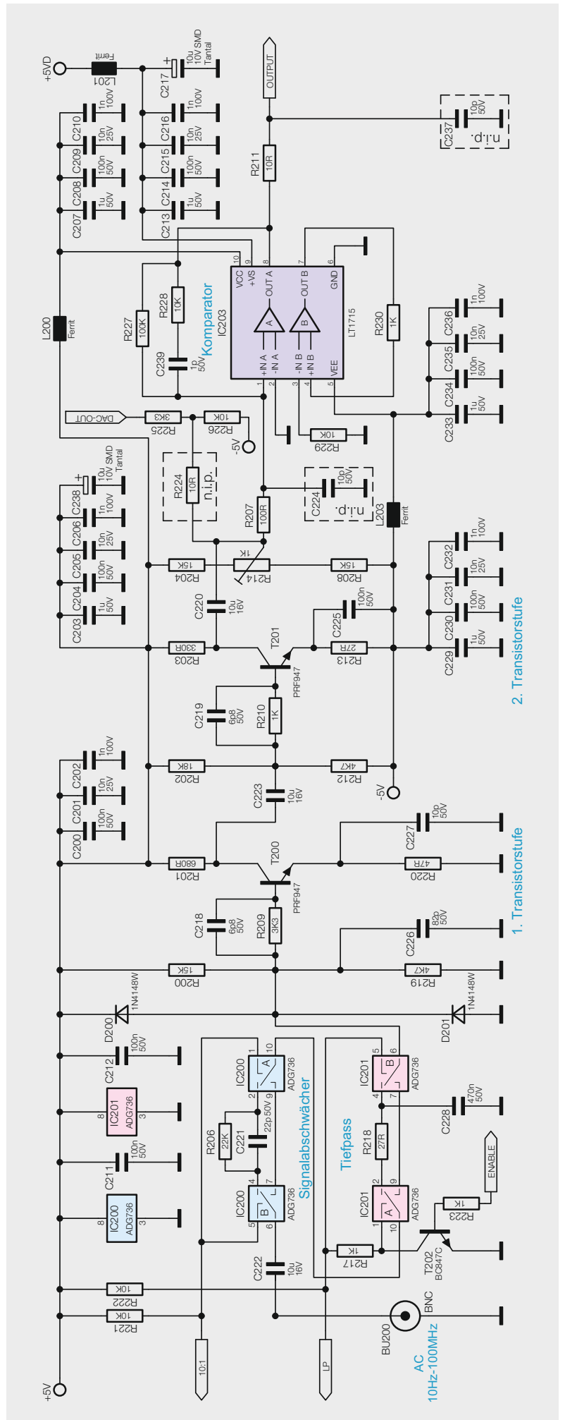
Bild 14: Das Schaltbild des Vorverstärkers für den Bereich 10 Hz bis 100 MHz
