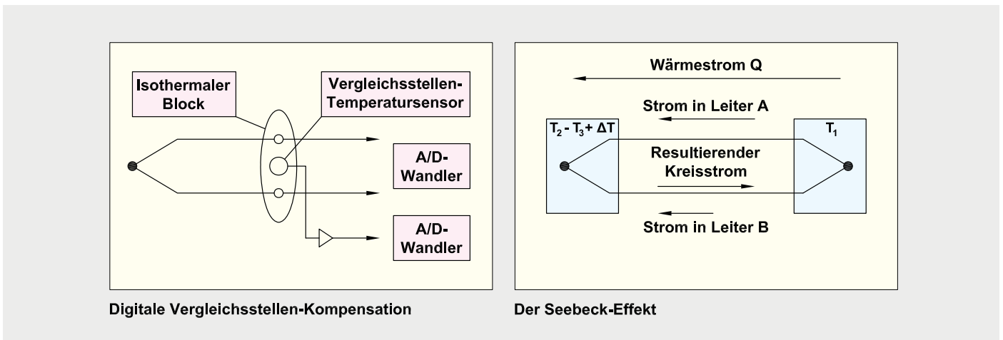
Bild 10: Digitale Kaltstellenkompensation und Seebeck-Effekt
