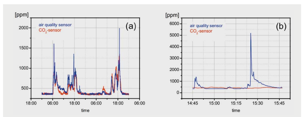
Bild 13: In einer nur gelegentlich frequentierten Toilette bewirkt ein einmaliges Geruchsereignis keinen CO 2 -Anstieg. ELV
