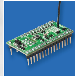
8-Kanal-Sendemodul
