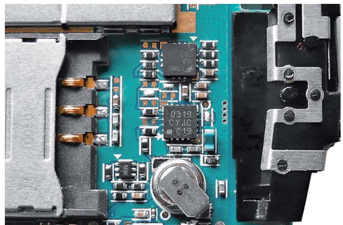
Einsatz des Si4703 in einem Smartphone. Man erkennt hier die minimale Außenbeschaltung, als Antenne dient die Zuleitung des Headsets.
