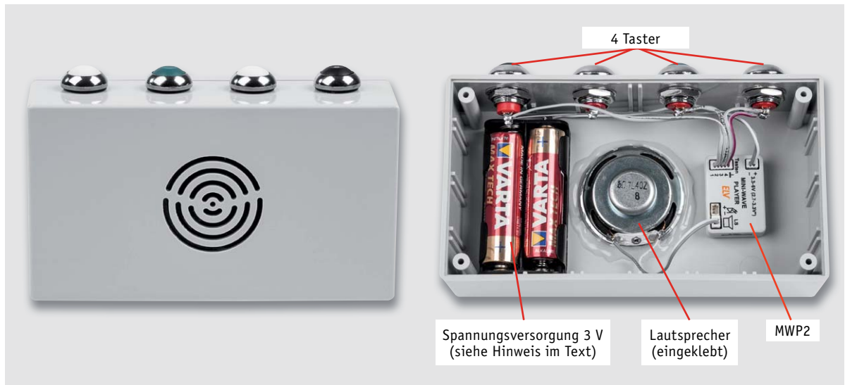
Bild 12: Beispiel für eine kleine Jingle-Box
