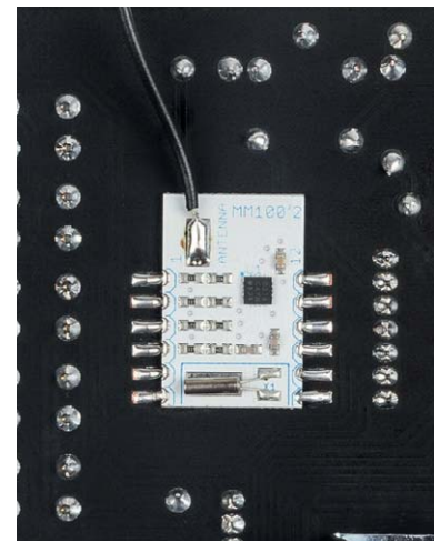
Bild 6: Hier ist die exakte Einbaulage des Empfängermoduls zu sehen.
