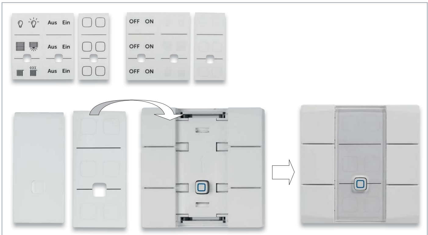
Bild 9: Zum Schluss erfolgt das Einlegen der Tastenbeschriftung. Vorlagen stehen zum Download bereit, anhand deren Maße kann man auch eigene Beschriftungen erstellen.
