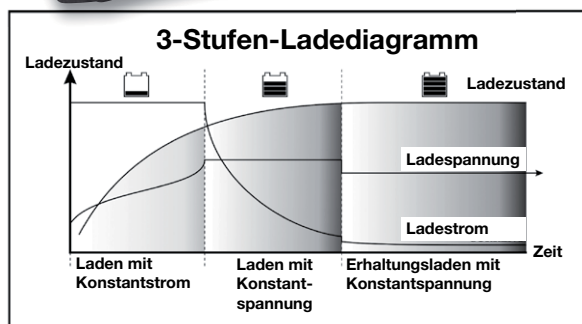
Bild 10: Mehr als nur ein Ladegerät, das 3-Stufen-Ladegerät Manson SBC-2110 mit zugehörigem IUoU-Ladediagramm. Bild: ELV
