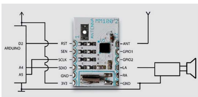
Bild 9: So erfolgt die prinzipielle Anbindung des Empfängermoduls an einen Arduino entsprechend der Si4703-Standard-Library.
