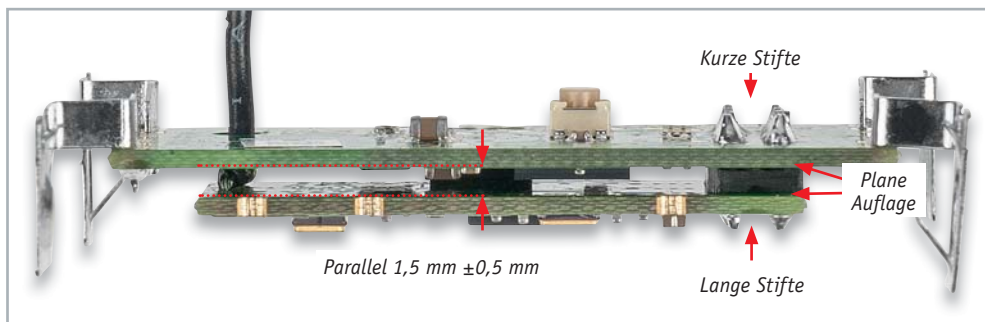
Bild 3: Das Funkmodul muss genau parallel zur Hauptplatine liegen.
