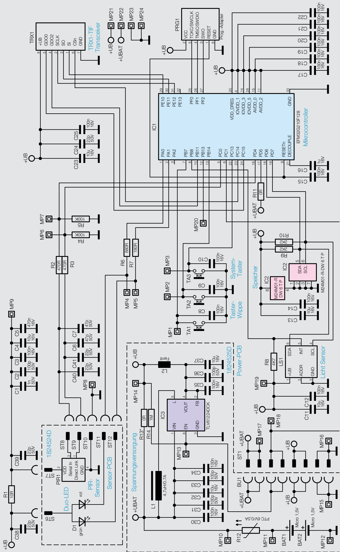
Bild 1: Das Schaltbild des HmIP-SMI55
