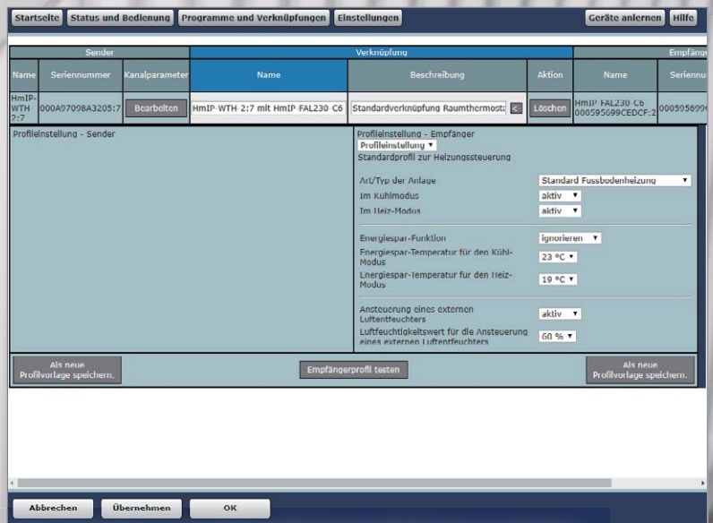
Bild 11: Einstellungen der direkten Verknüpfung (Verknüpfung bearbeiten)
