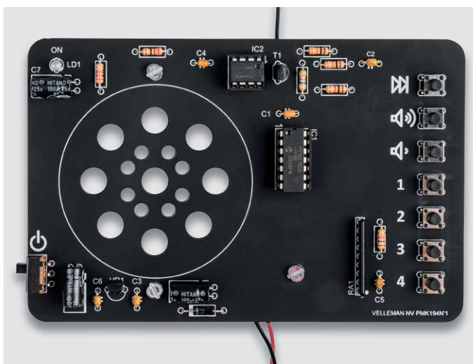
Bild 7: Die vollständig bestückte Vorderseite des Radio-Bausatzes
