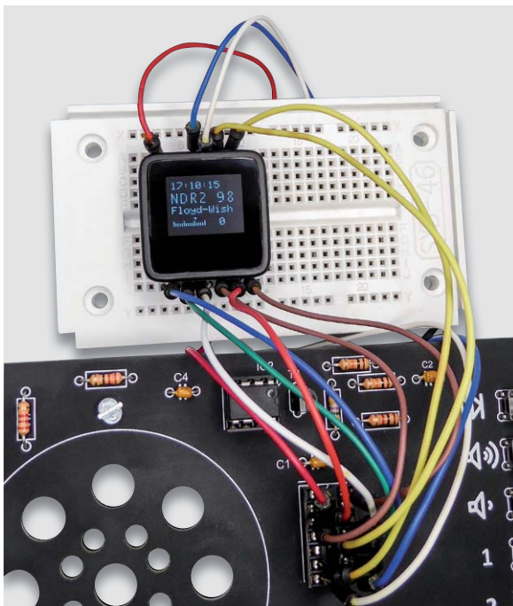
Bild 14: Der MicroView am Radiobausatz in Aktion. Das OLED-Display erlaubt eine scharfe Darstellung auch kleiner Schriften und Grafiken.
