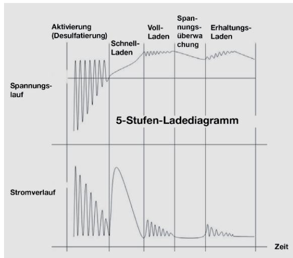
Bild 9: Typisches Ladediagramm für ein modernes, intelligentes Ladegerät
