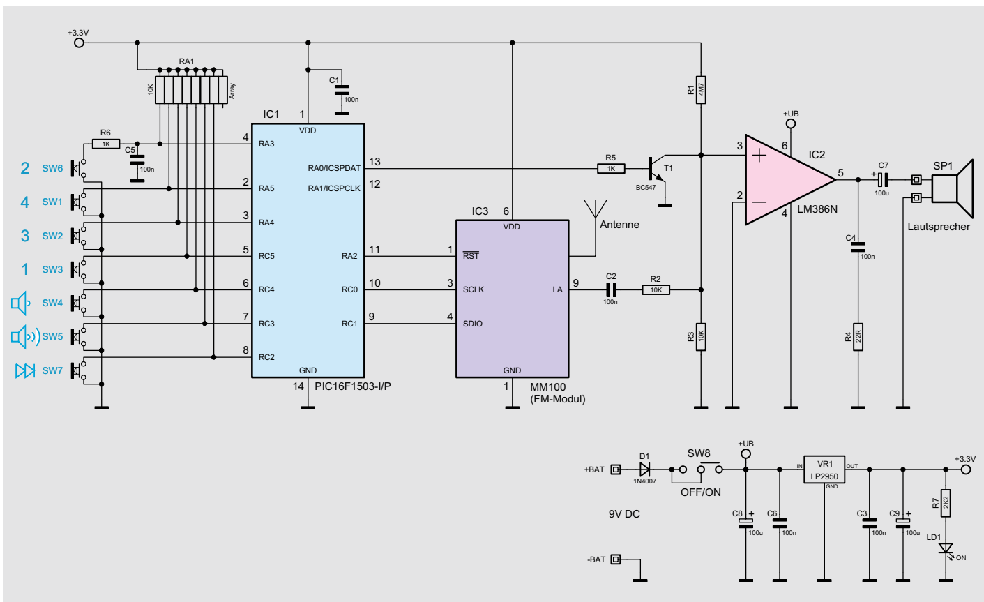
Bild 3: Das Schaltbild des MK194N
