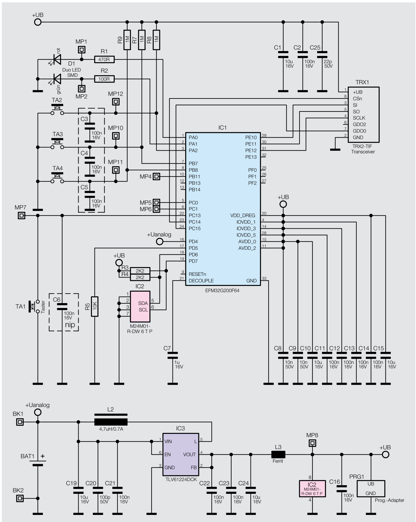
Bild 2: Das Schaltbild des Fenstergriffsensors HmIP-SRH
