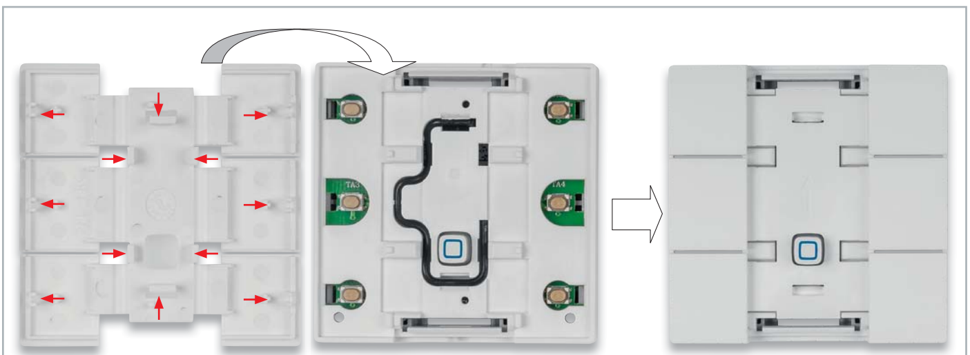
Bild 8: Beim Aufstecken der Tastereinheit ist darauf zu achten, dass die insgesamt 12 Rasten sauber einrasten.
