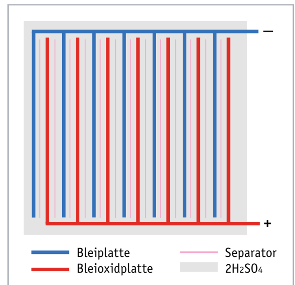
Bild 1: Der Aufbau eines 12-V-Blei-Säure-Akkus
