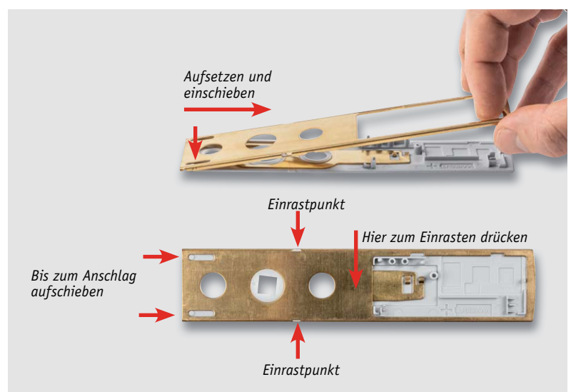
Bild 6: Die Metallabdeckung ist wie hier gezeigt aufzuschieben, einzulegen und einzurasten.
