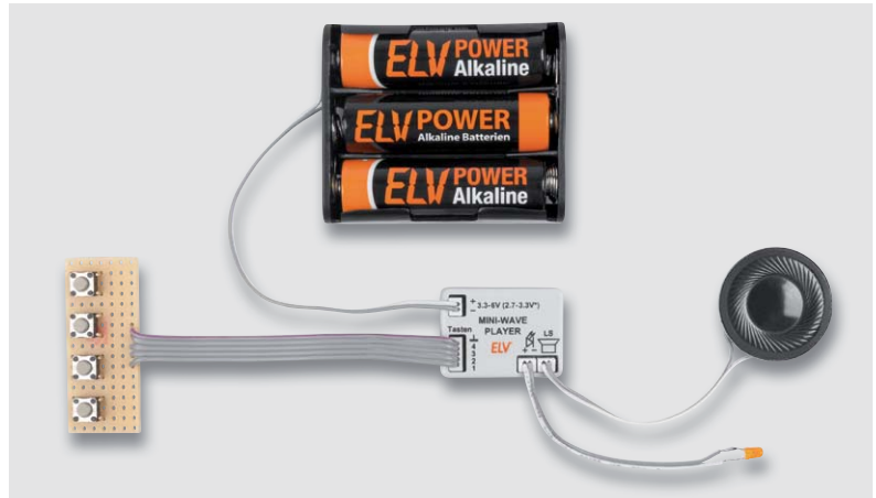
Bild 6: Anwendungsbeispiel mit Batteriebetrieb
