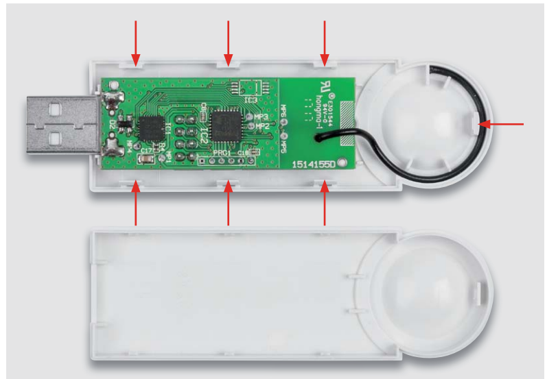
Bild 5: Die Antenne ist wie hier gezeigt in den Antennenhalter einzulegen. Hier sind auch die Gehäuseersten für das spätere Zusammsetzen der Gehäuseteile markiert.
