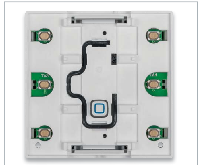
Bild 7: So wird die Antenne in die dafür vorgesehene Gehäuseaussparung eingelegt.
