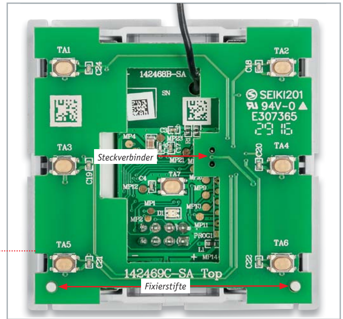
Bild 5: Beim Aufstecken der Tasterplatine ist anhand des Steckverbinders und der Fixierstifte auf die richtige Lage zu achten.
