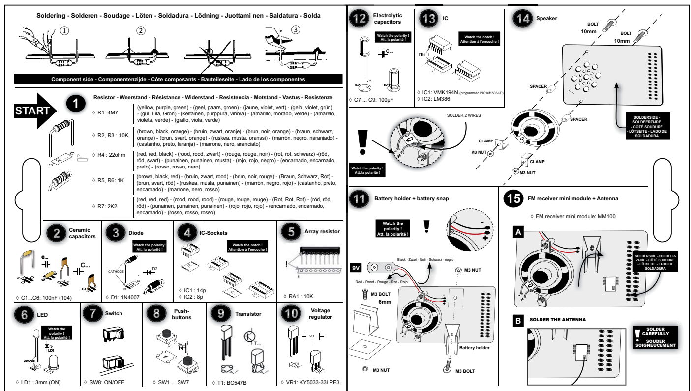
Bild 5: Die Bauanleitung des Bausatzes
