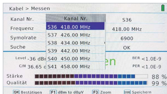
Bild 32: Voreingestellte Liste der Kanalbezeichnungen und -frequenzen
