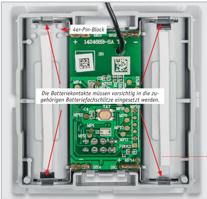
Bild 4: So erfolgt das Einlegen der Hauptplatine in das Gehäuseunterteil.
