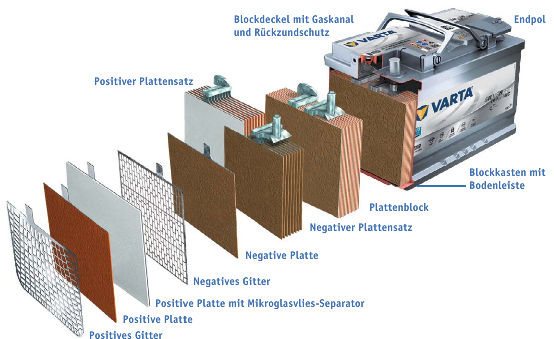
Bild 6: Beim AGM-Akku ist das Elektrolyt in einem Mikroglasvlies-Separator gebunden. Bild: Varta
