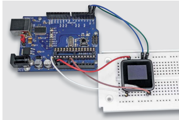
Bild 13: Eine Arduino-UNO-Platine als Programmier-Interface für den MicroView
