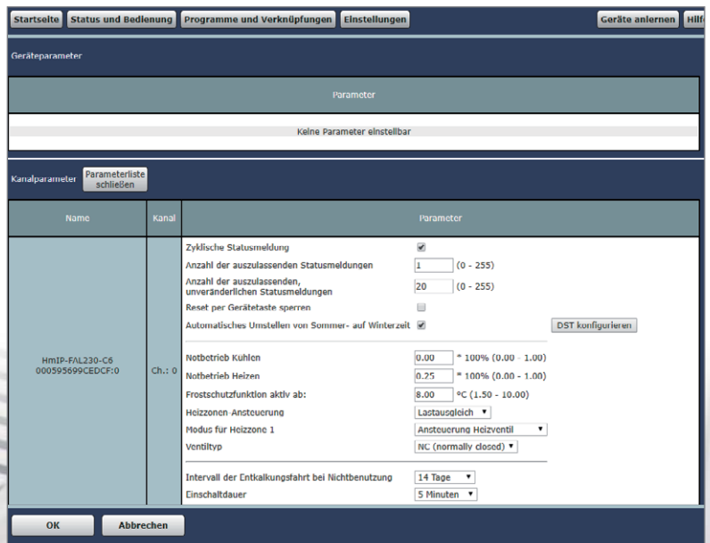
Bild 10: Ausschnitt der Geräteparameter der HmIP-FAL
