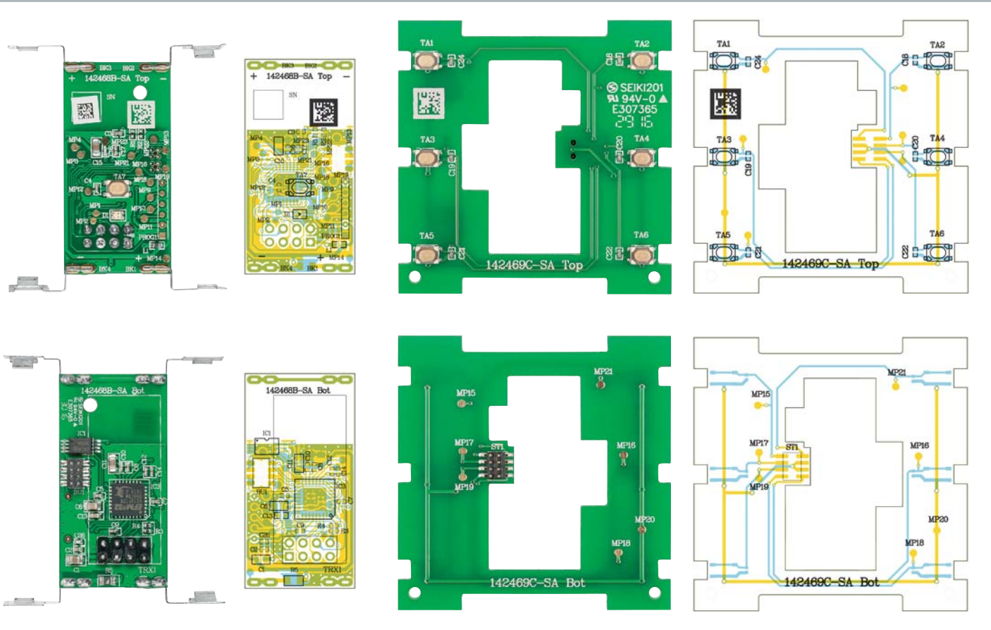
Bild 2: Die Platinenfotos und Bestückungspläne des HmIP-WRC6, links die Hauptplatine, rechts die Tasterplatine
