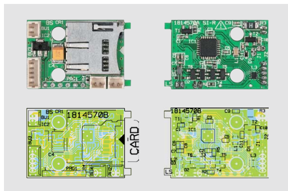
Bild 3: Fertig aufgebaute Platine mit zugehörigem Bestückungsplan, von der Bestückungsseite (links) und der Lötseite (rechts) gesehen
