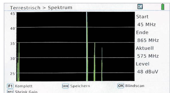
Bild 24: Im Test wurden auf drei Kanälen DVB-T2-Bouquets mit je fünf öffentlich-rechtlichen Programmen gefunden.
