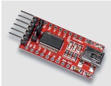
Bild 11: Über den speziellen Programmieradapter ist der MicroView bequem per Arduino-IDE zu programmieren.
