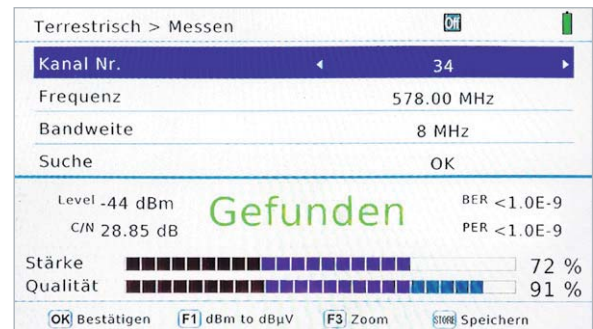
Bild 22: Bei einem erfolgreichen Suchlauf nach einem DVB-T/T2-Sender erscheint der grüne Schriftzug „Gefunden“ und die damit zusammenhängenden Messwerte.
