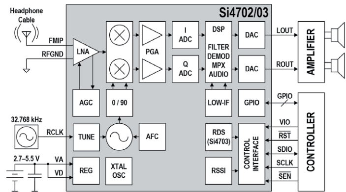
Das Blockschaltbild des Si4703, eingebettet in eine komplette Empfängerkonfiguration
