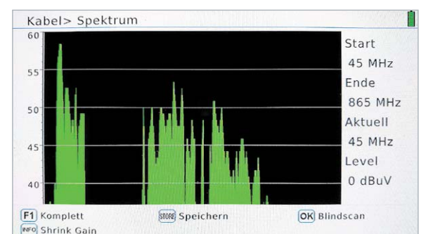
Bild 35: Das komplette Kabelspektrum zwischen 45 und 865 MHz mit starken Pegelschwankungen
