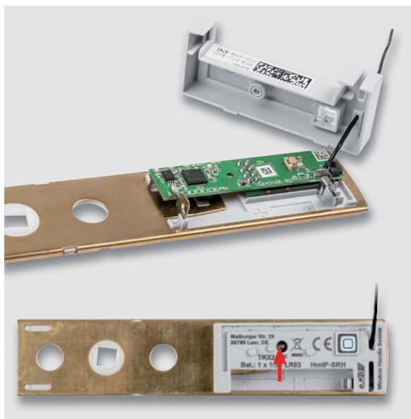
Bild 9: Nach dem Durchführen der Antenne durch das Elektronikgehäuse (oben) wird dieses aufgesetzt und mit einer Schraube vorsichtig verschraubt (unten).
