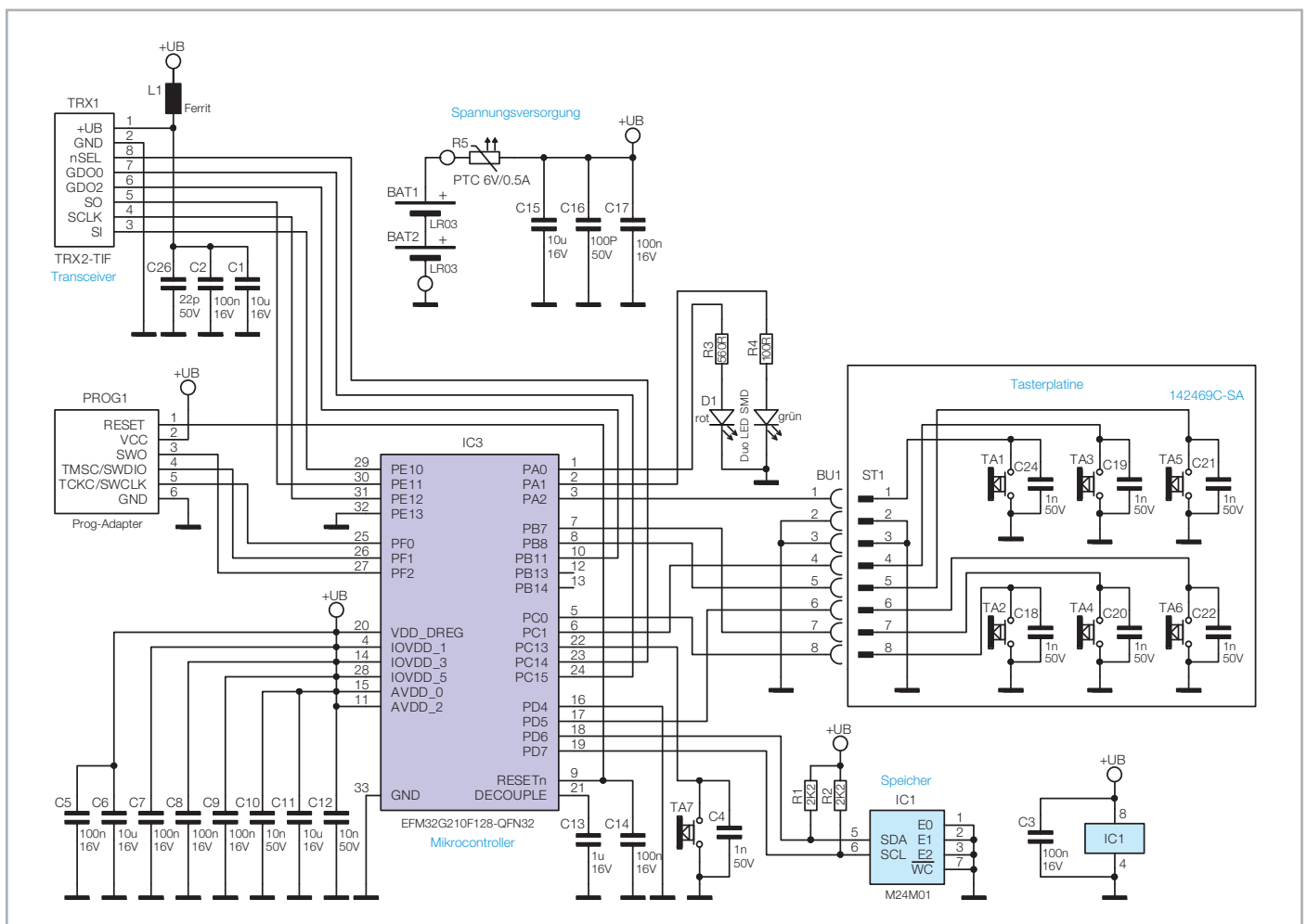
Bild 1: Das Schaltbild des Homematic IP 6fach Funk-Wandtasters
