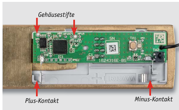
Bild 8: So liegt die Platine exakt im Gehäuse: Die Gehäusestifte ragen durch die Platine und die Batteriekontakte in den dafür vorgesehenen Halter.
