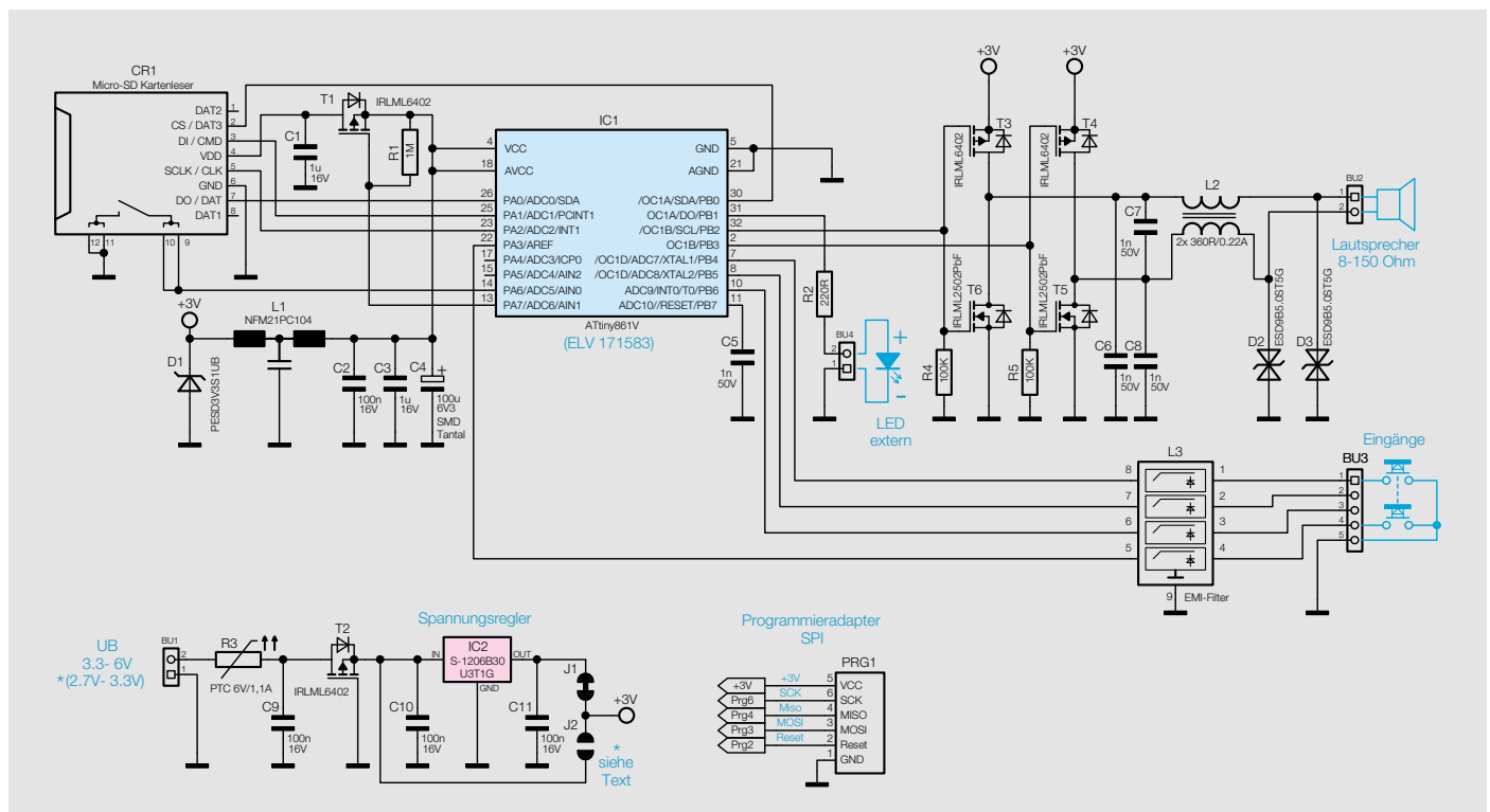
Bild 2: Schaltbild des Mini-Wave-Players
