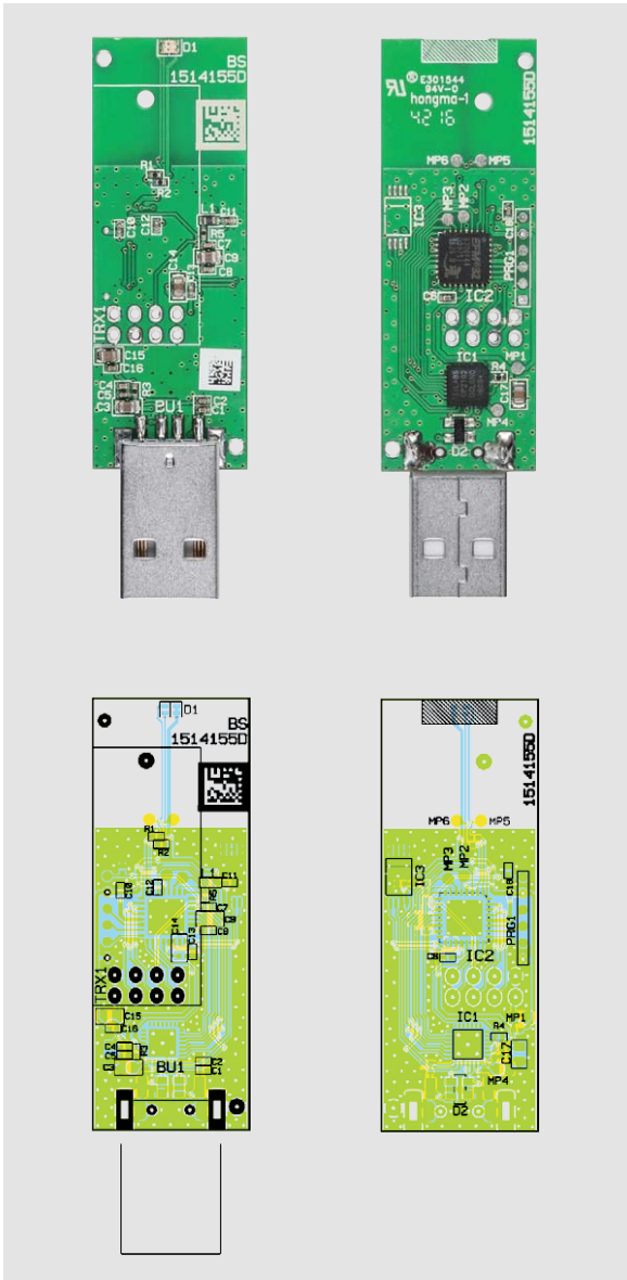
Bild 3: Platinenfotos sowie die zugehörigen Bestückungspläne der Platine
