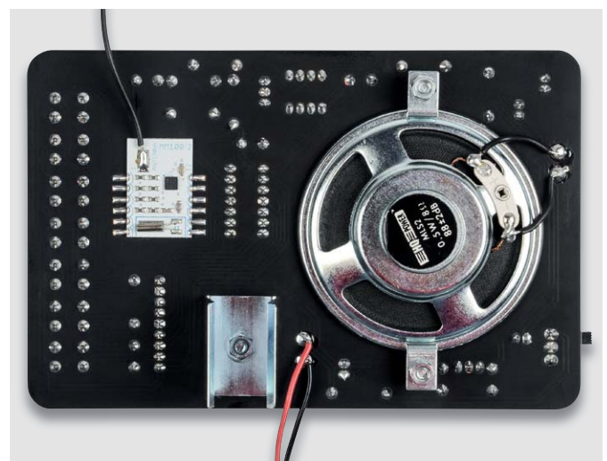
Bild 8: Die vollständig bestückte Rückseite des Radio-Bausatzes
