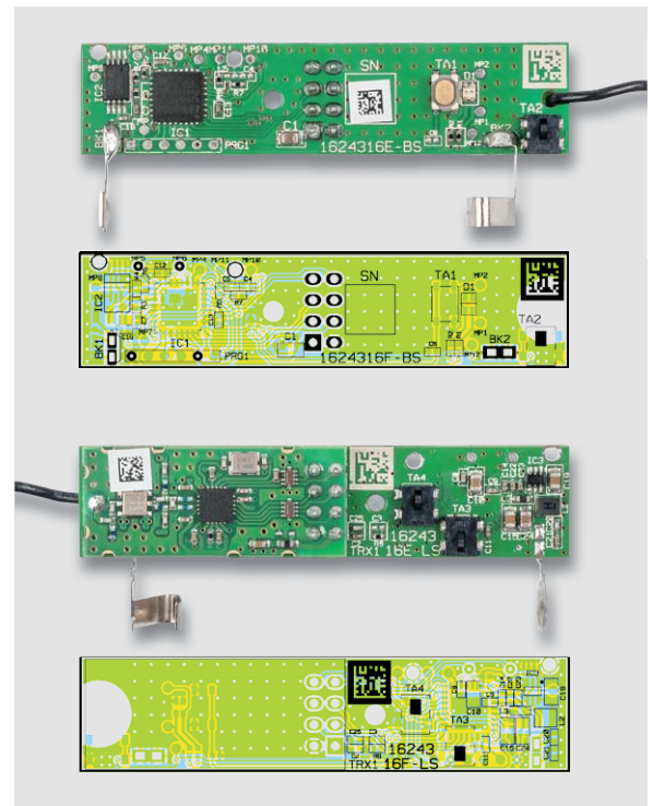
Bild 3: Die Platinenfotos der komplett bestückten Platine mit den zugehörigen Bestückungsplänen
