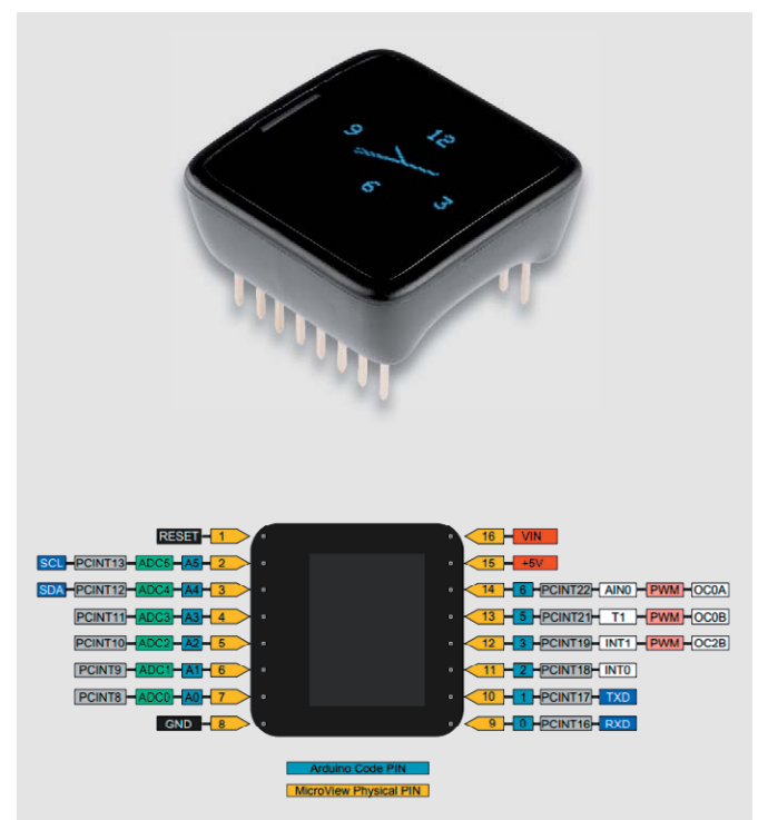
Bild 10: Der MicroView in Aktion, daneben sein Pinout und der Pin-Bezug zu den Arduino-Standard-Anschlüssen
