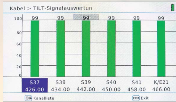
Bild 37: „Kabel > TILT Signalauswertung“ veranschaulicht die Schräglage (Pegeldifferenz) innerhalb einer Gruppe von sechs benachbarten Kanälen. Sie soll möglichst gering sein.
