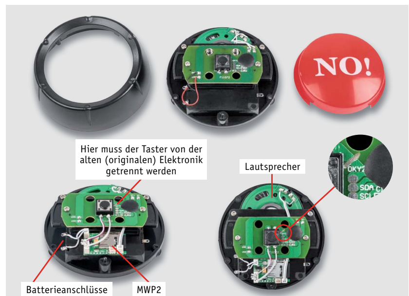
Bild 16: Original und umgebaute Variante eines Sound-Buttons
