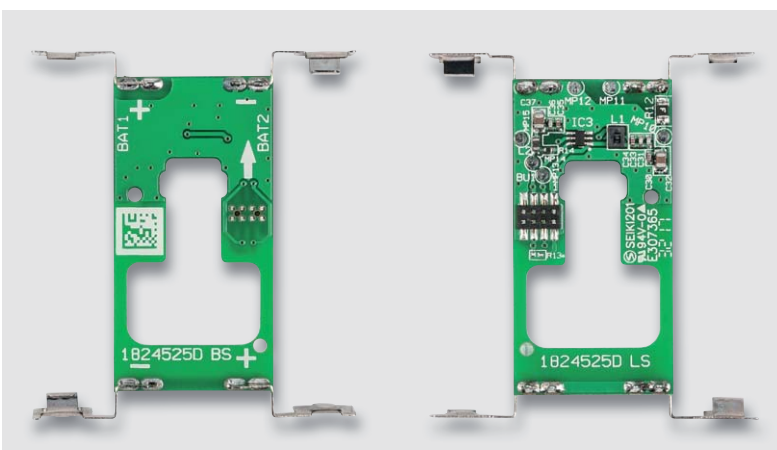
Bild 3: Die Batterieplatine mit den bestückten Batteriekontakten
