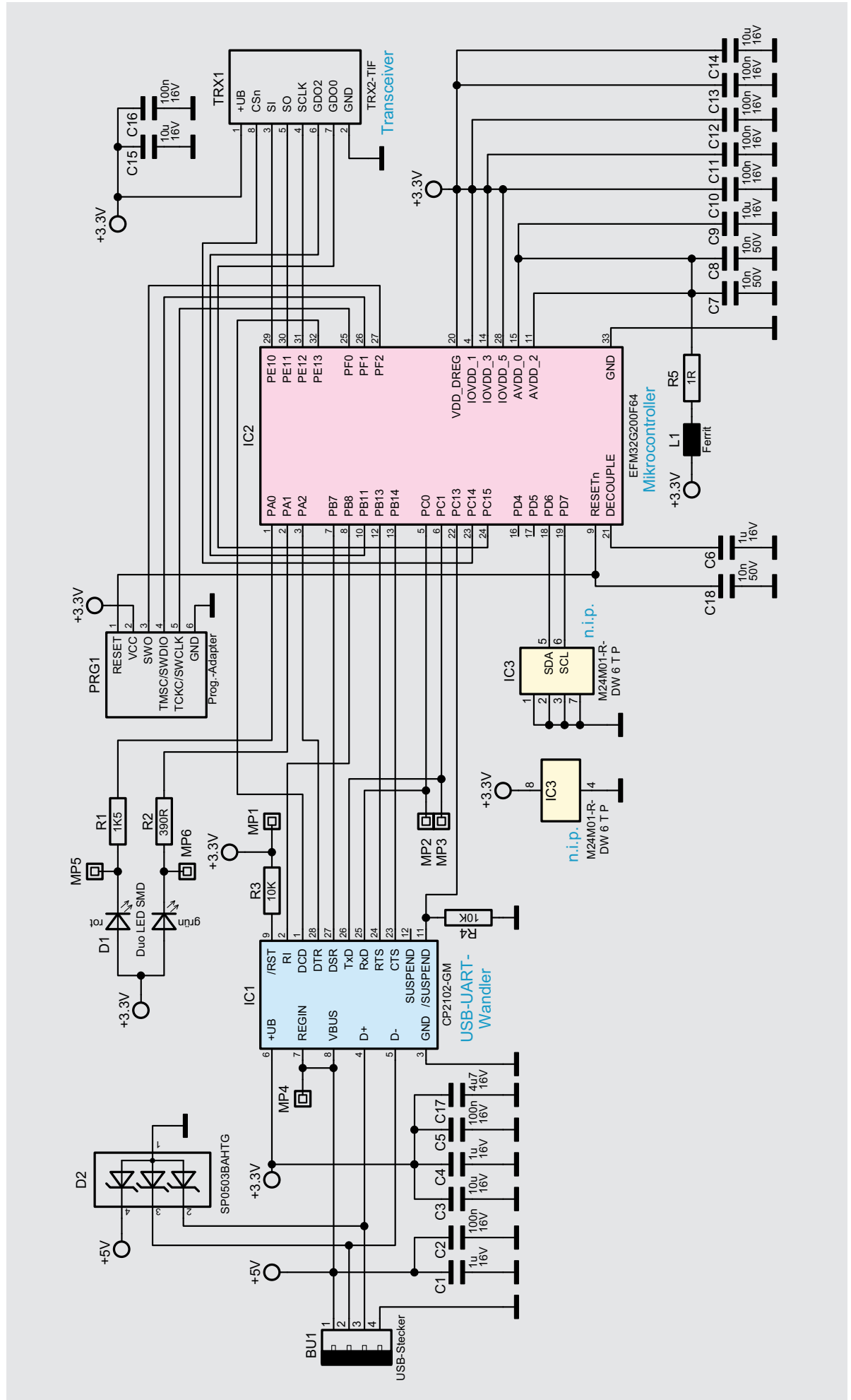
Bild 1: Das Schaltbild des HmIP-RFUSB
