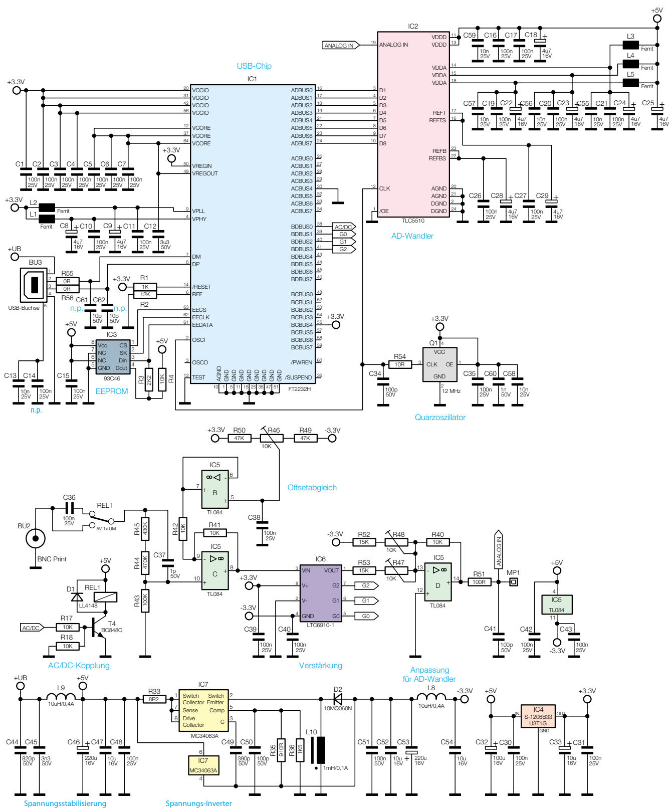
Bild 2: Das Schaltbild des USB-MSM
