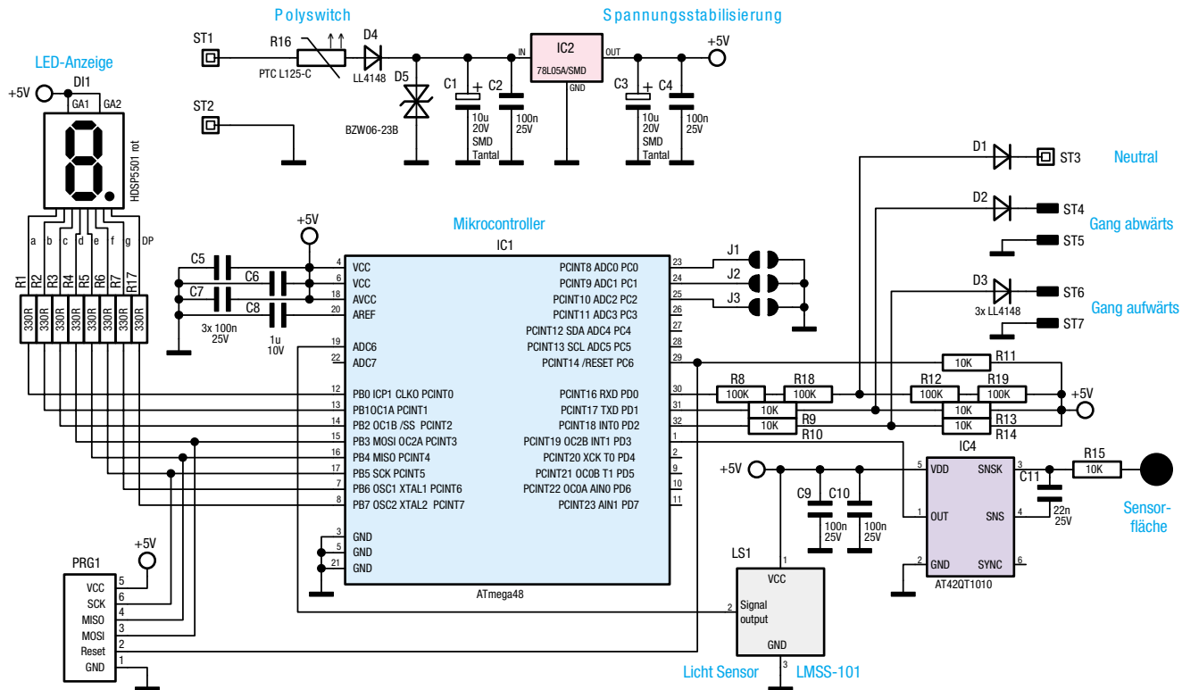
Bild 1: Schaltbild der Motorrad-Ganganzeige
