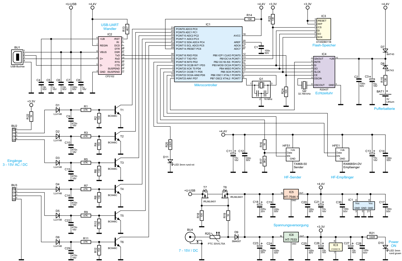
Bild 5: Das Schaltbild der FS20 MST2
