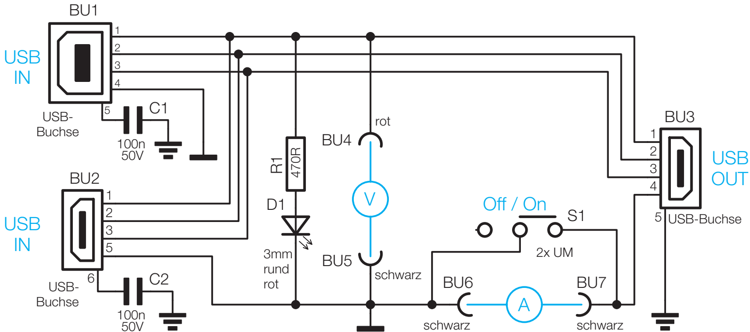
Das Schaltbild des USB-Messadapters
