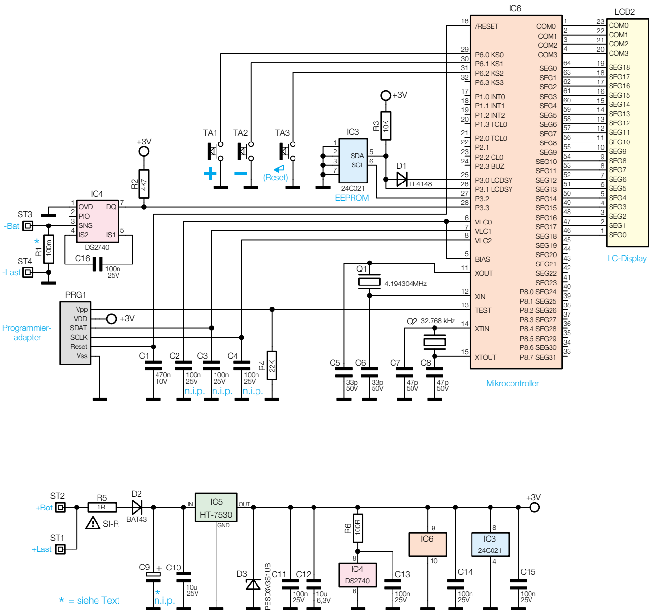
Bild 2: Das Schaltbild des GZM 100
