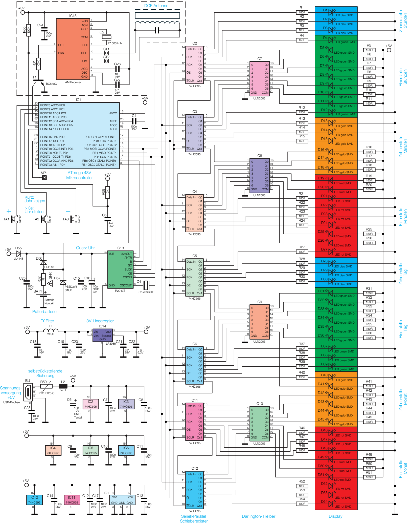
Das Schaltbild der Binäruhr B2
