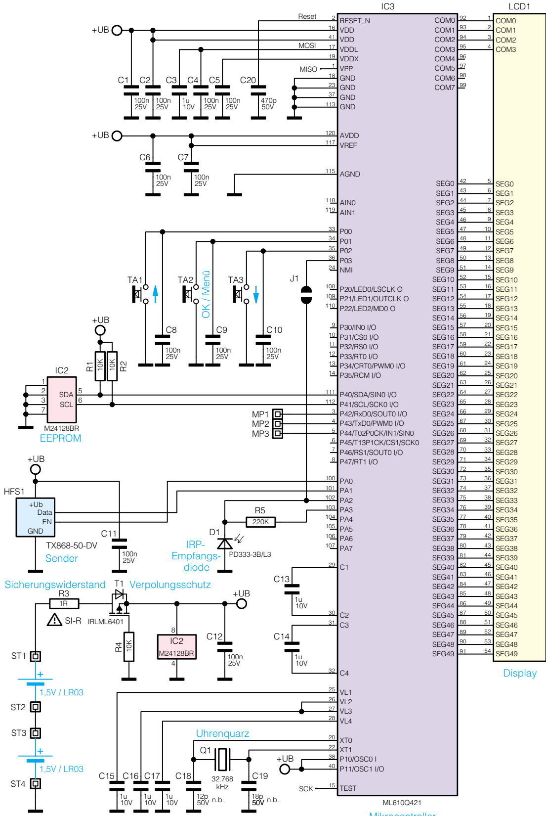
Bild 4: Das Schaltbild der FS20 ZSU
