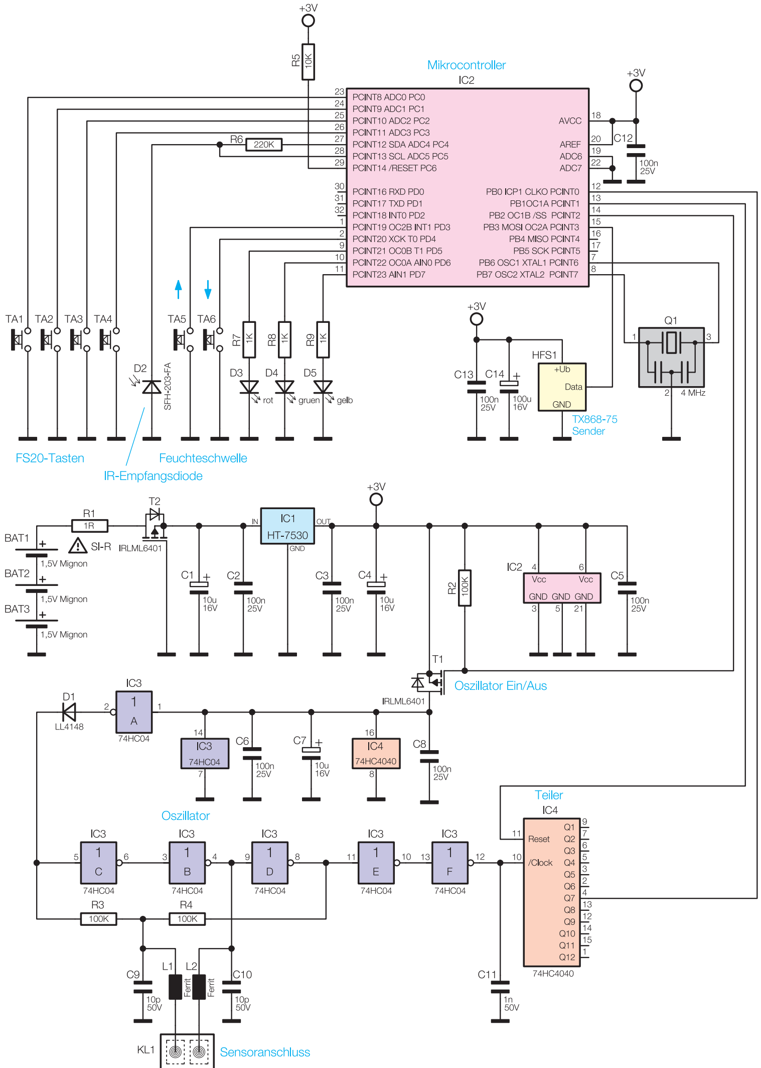
Schaltbild des FS20-Bodenfeuchtesensors
