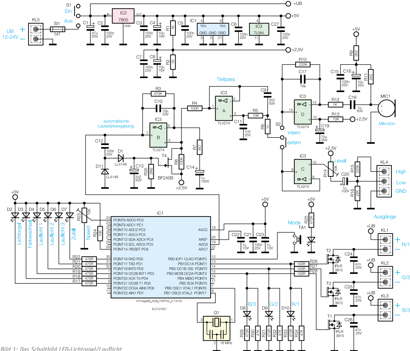
Bild 1: Das Schaltbild LED-Lichtorgel/Lauflicht
