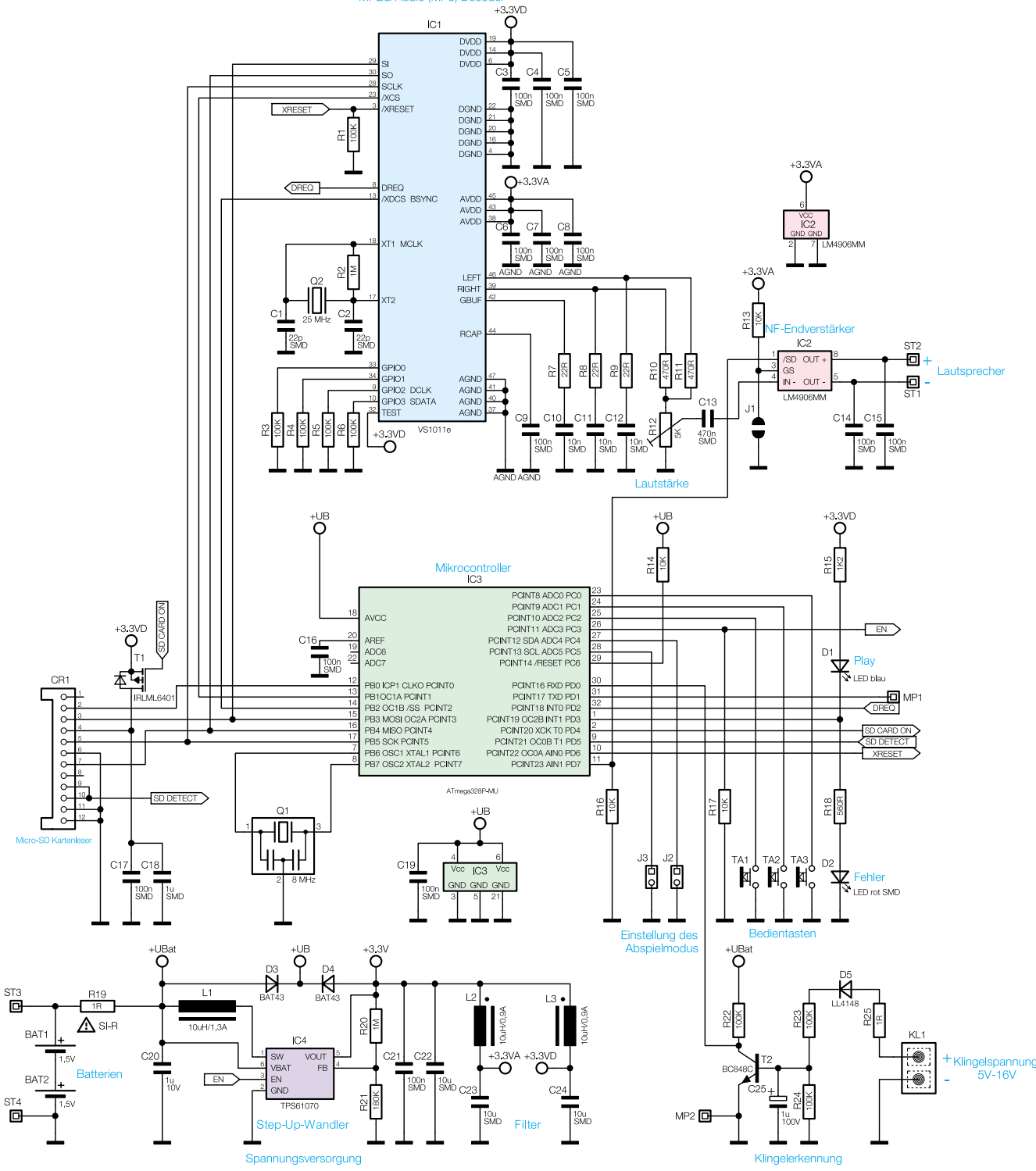
Bild 2: Schaltbild der MP3-Türklingel
