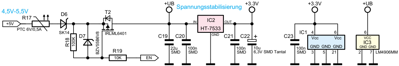
Bild 9: Spannungsversorgung des MSM 2
