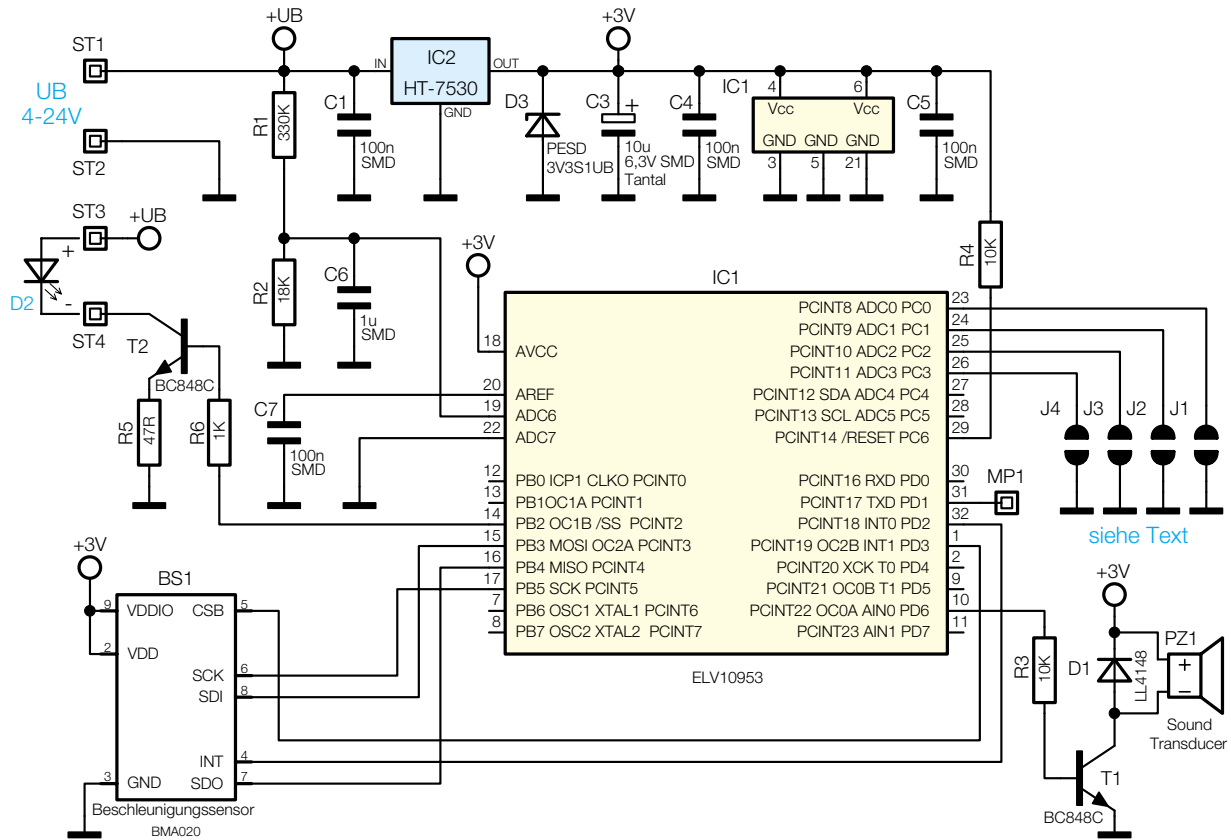
Bild 3: Schaltbild des Ortungspiepers
