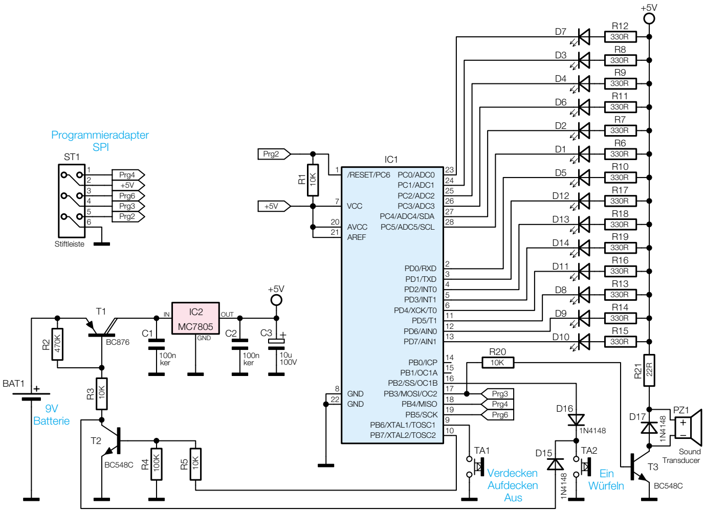
Bild 1: Die Schaltung des Würfelspiels, minimalistisch dank Mikrocontroller
