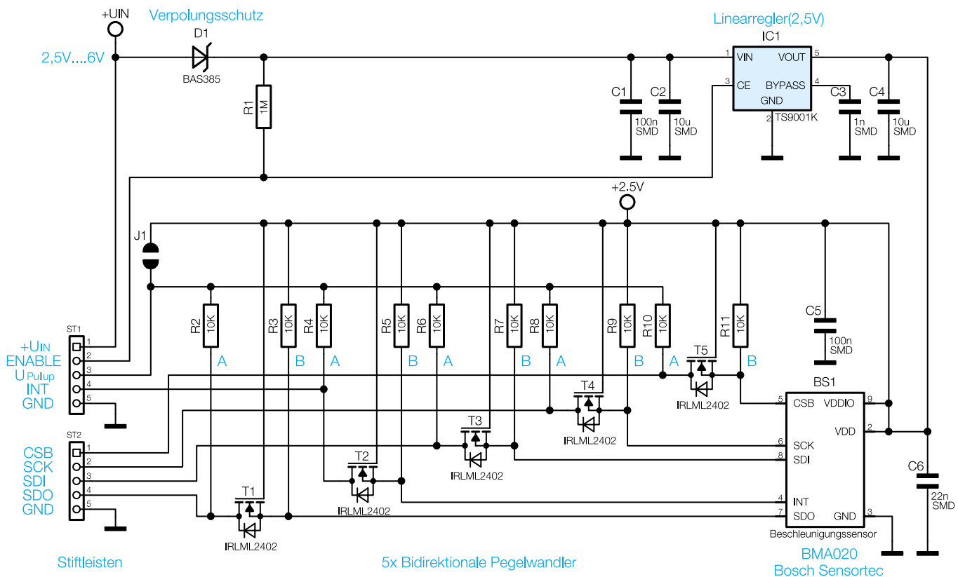
Bild 6: Schaltplan des 3D-BS-Moduls
