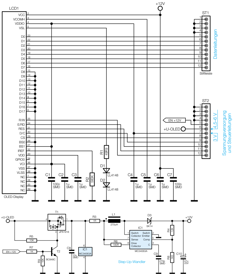
Bild 2: Schaltung des OLED-Displaymoduls
