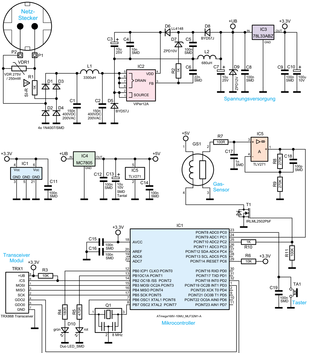
Bild 4: Die Gesamtschaltung des CO 2 -Sensors
