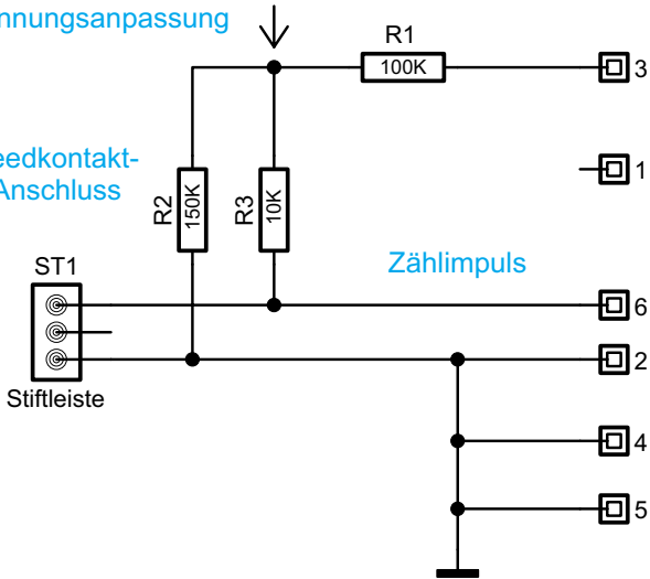
Bild 6: Schaltbild der Interfaceplatine
