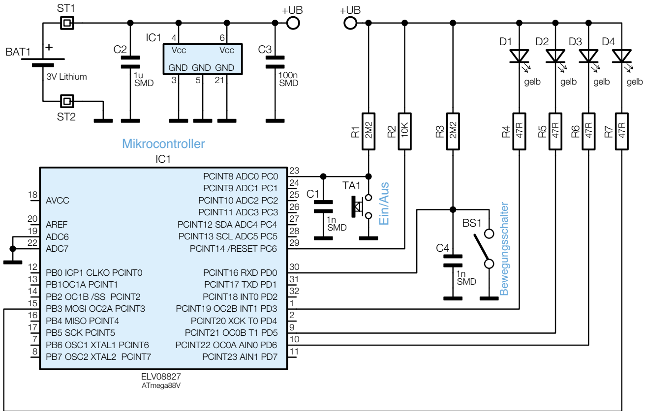
Bild 1: Das Schaltbild des LED-Kerzenlichts
