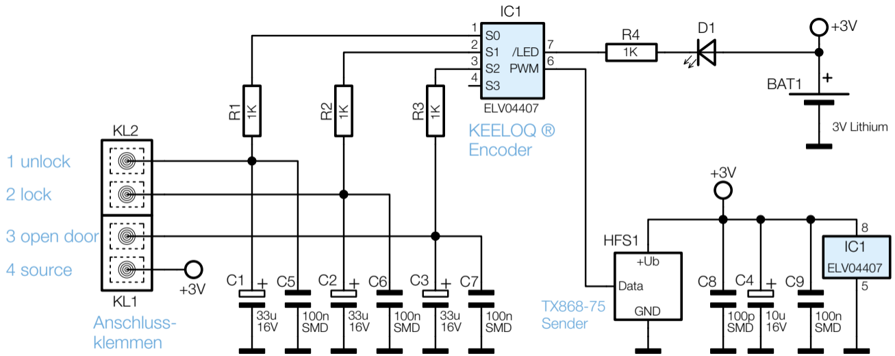
Bild 1: Das Schaltbild des KM300 PBI
