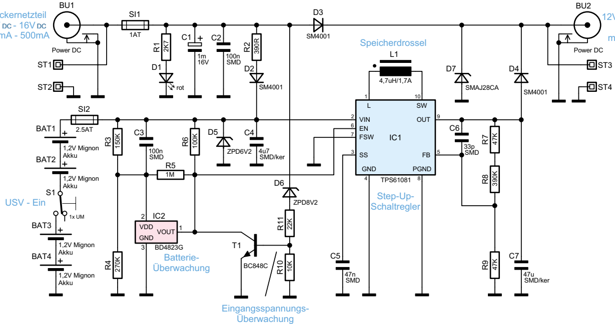
Bild 2: Schaltbild der unterbrechungsfreien Stromversorgung USB 12
