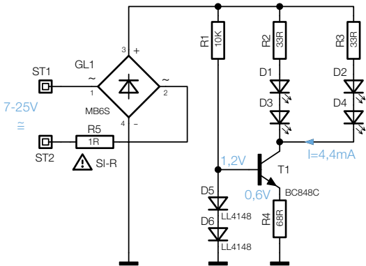
Bild 3: Die Schaltung der LED-Ansteuerung
