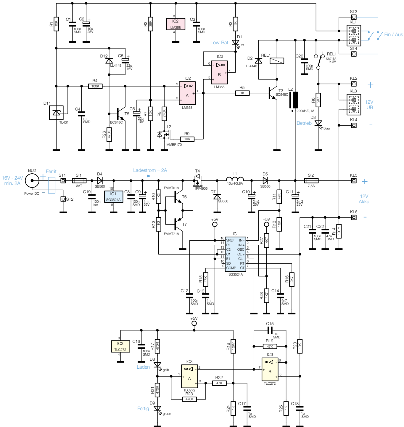
Bild 6: Das Schaltbild der Ladeschaltung
