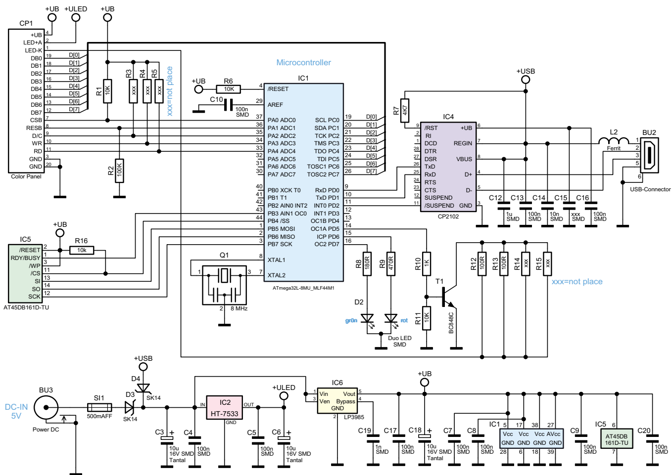
Bild 2: Die Schaltung des LCP 100
