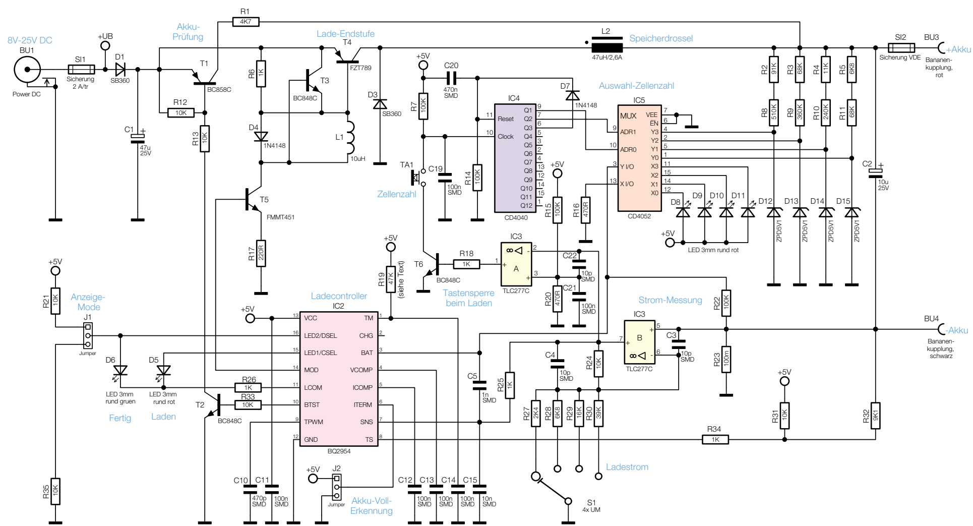
Bild 4: Hauptschaltbild des LiFe 4
