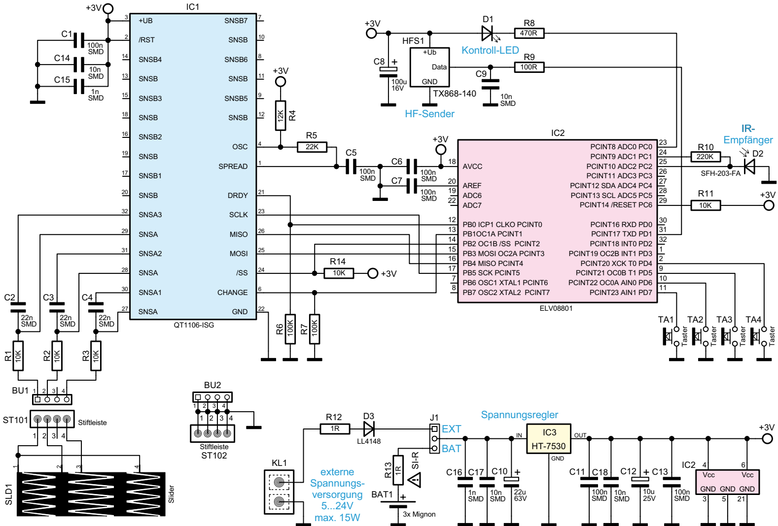
Bild 4: Schaltbild des FS20-Dimmer-Sliders
