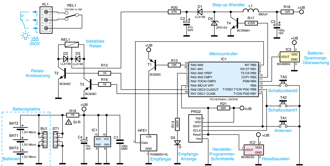
Bild 1: Schaltbild des KeyMatic®-Schaltaktors KM300 SB
