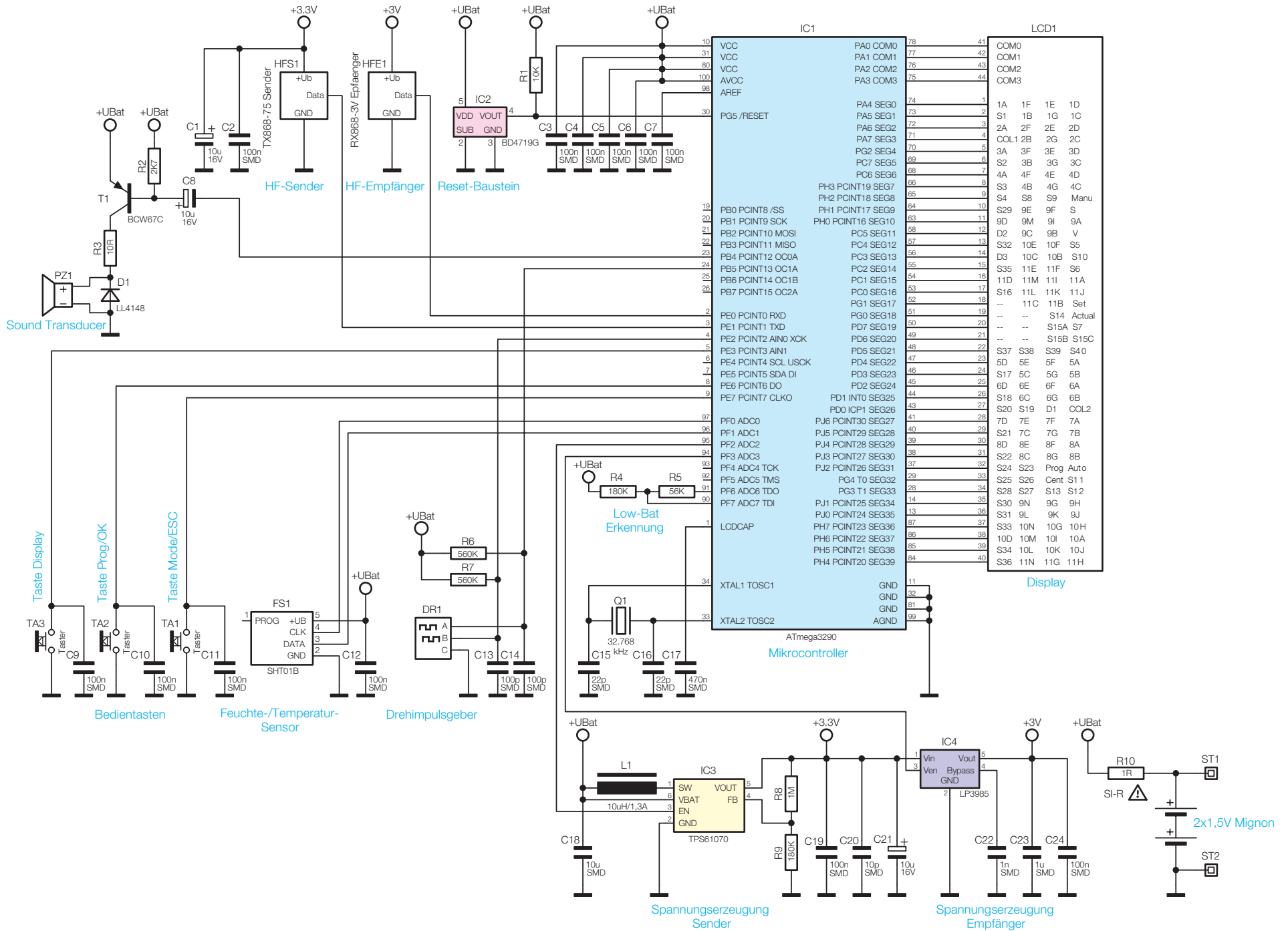
Bild 2: Das Schaltbild der FS20 LES
