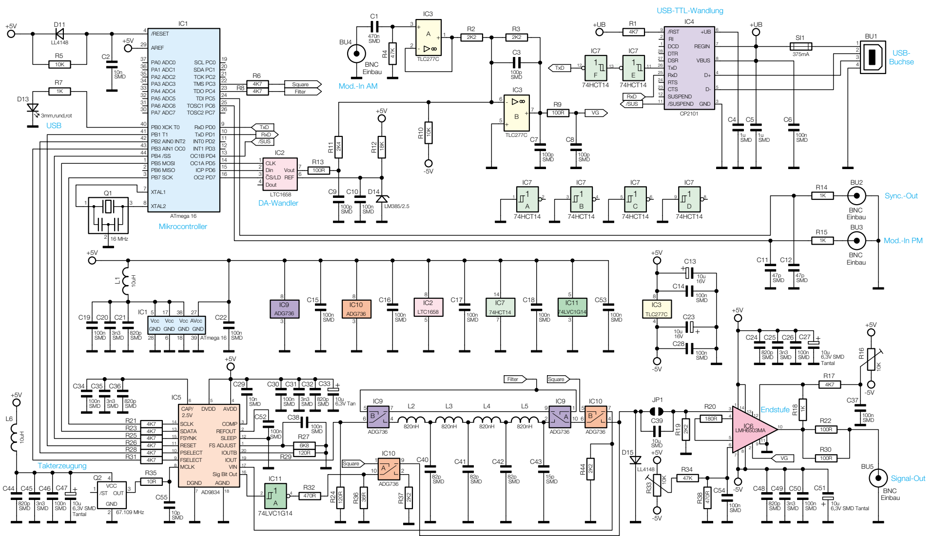
Bild 2: Das Schaltbild des DDS 130
