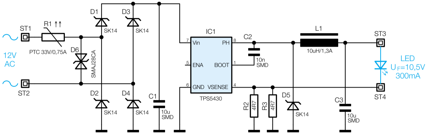
Bild 2: Die Ansteuerschaltung für die 3-W-Flächen-LED
