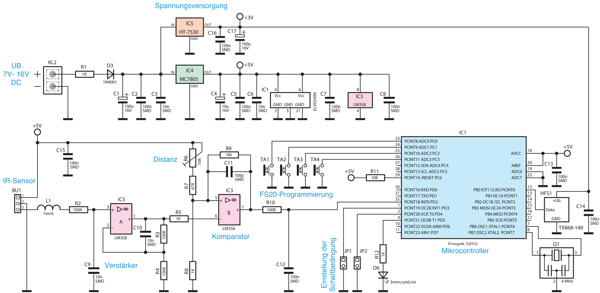
Bild 4: Das Schaltbild der FS20 OE
