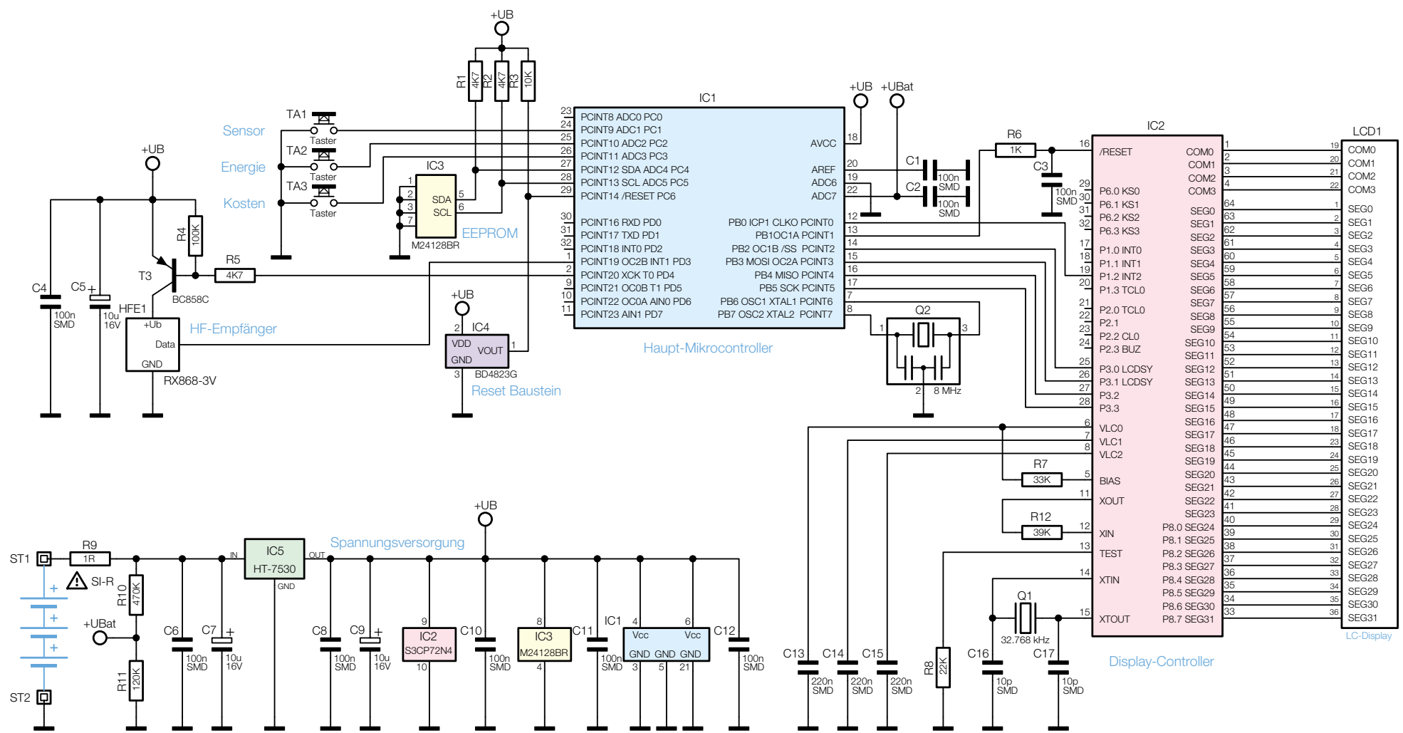
Bild 4: Das Schaltbild der ESA 1000
