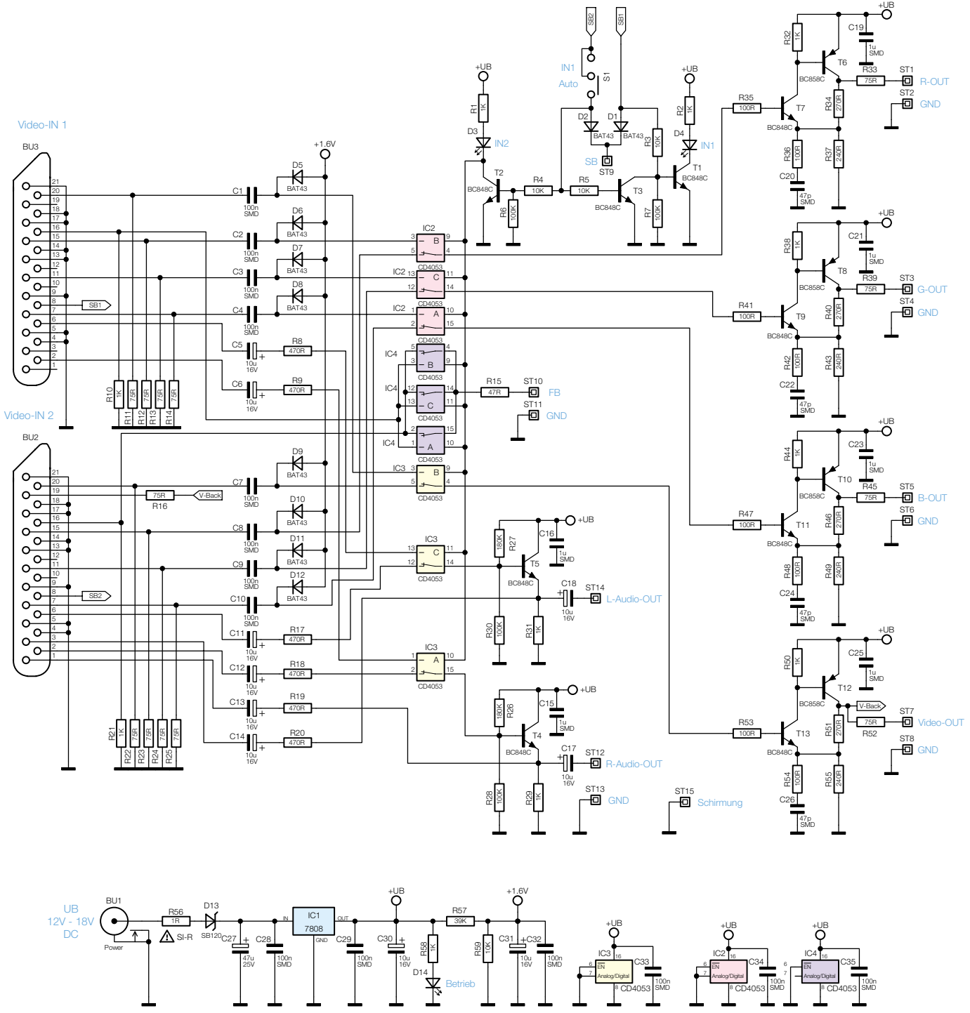
Bild 2: Schaltbild des AVS 2
