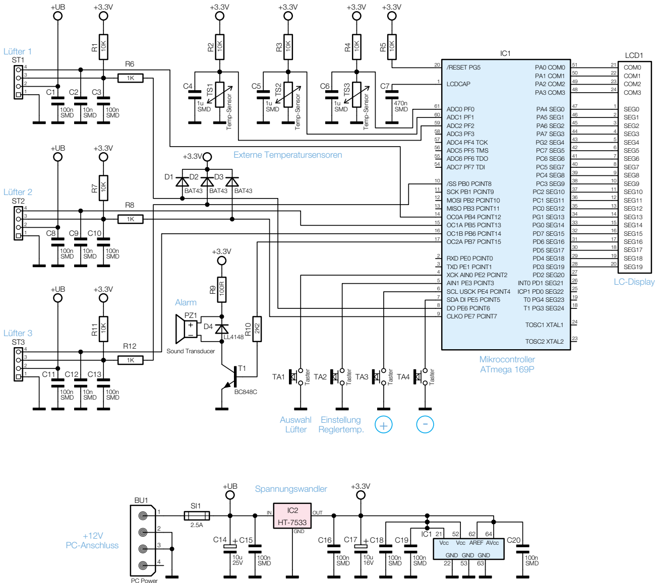
Bild 5: Das Schaltbild der PLS 100
