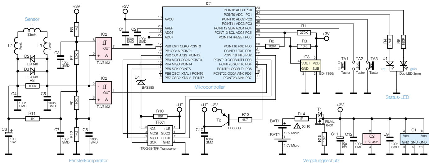
Bild 13: Das Schaltbild des HM-Sen-EP
