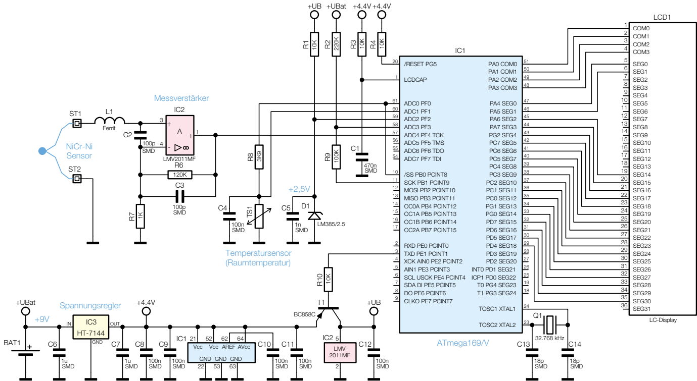
Bild 2: Schaltbild des Lötcolbentemperatur-Messgerätes
