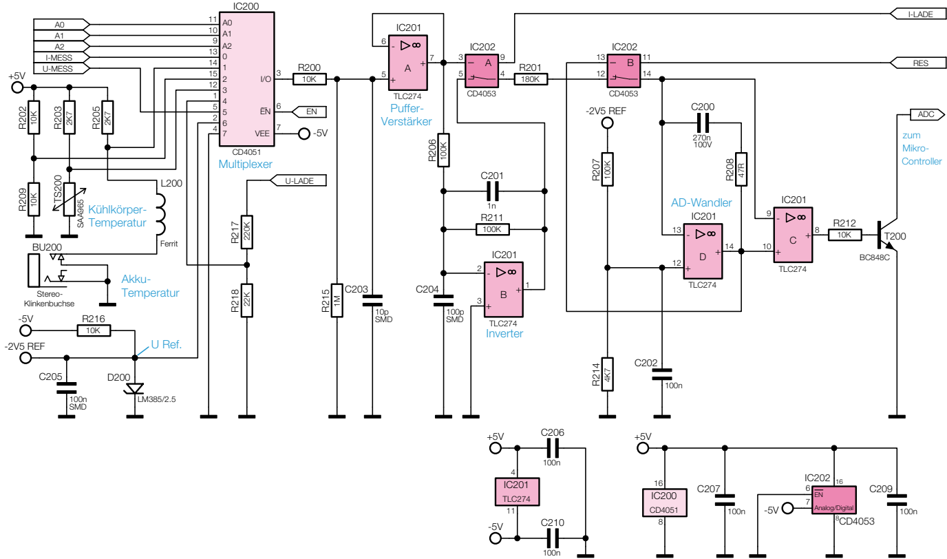
Bild 8: Analog-Digital-Wandler des ALC 3000 PC
