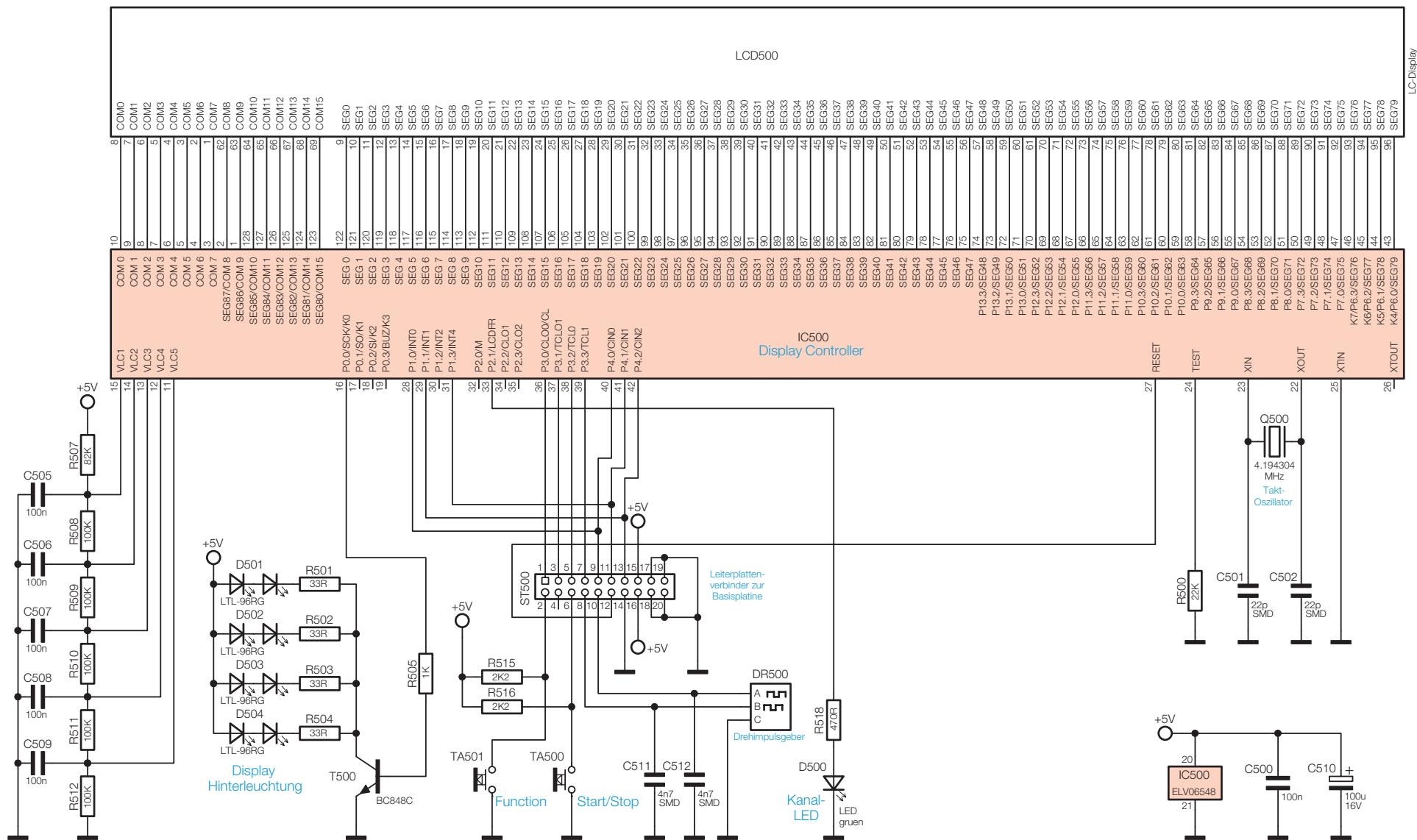
Bild 6: Displayeinheit des ALC 3000 PC
