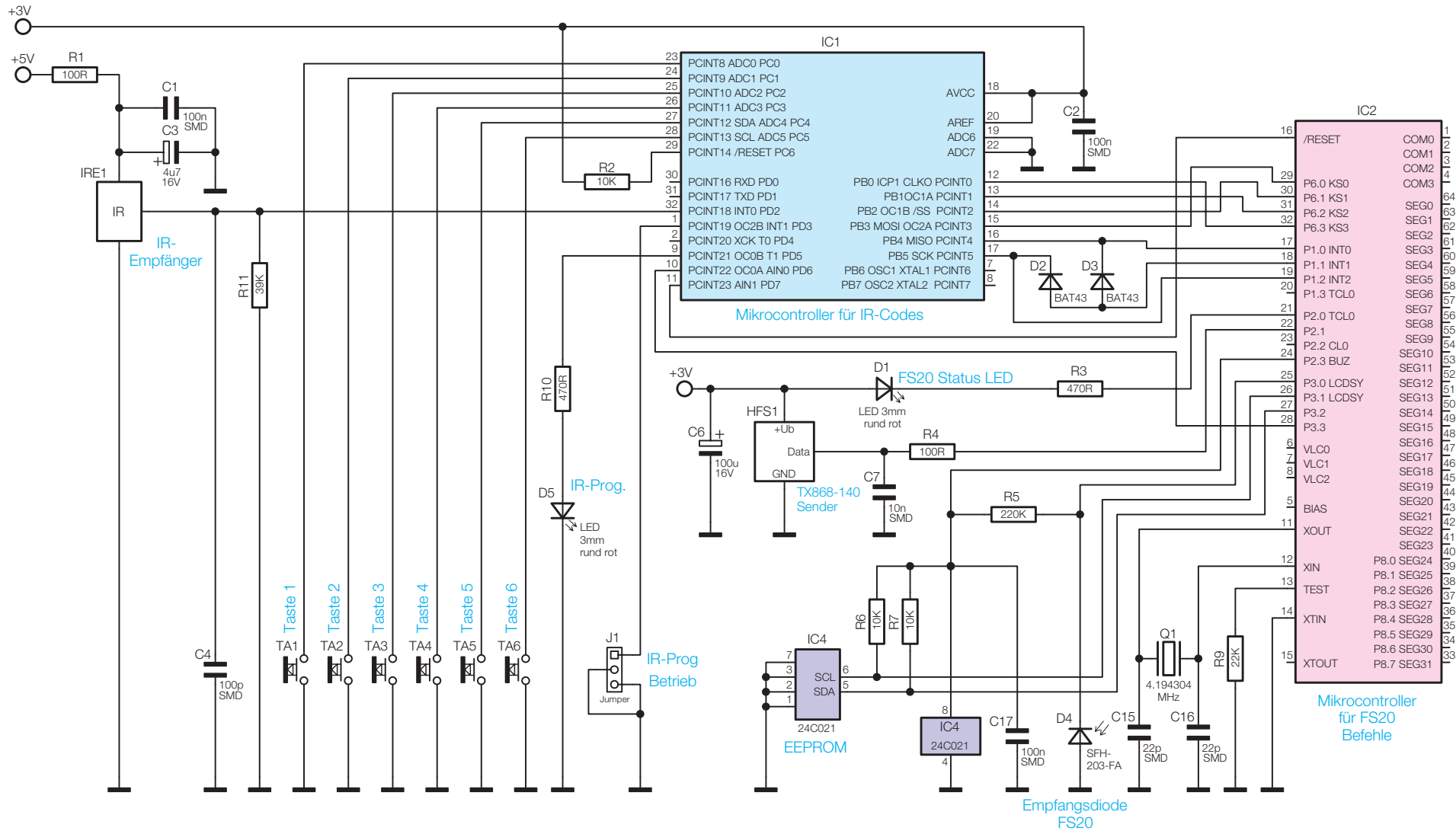
Bild 13: Schaltung des FS20 IRU
