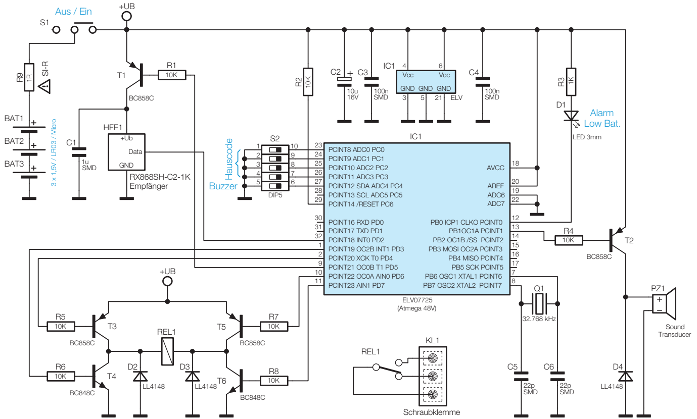
Bild 1: Schaltbild des Funk-Rauchalarm-Empfängers
