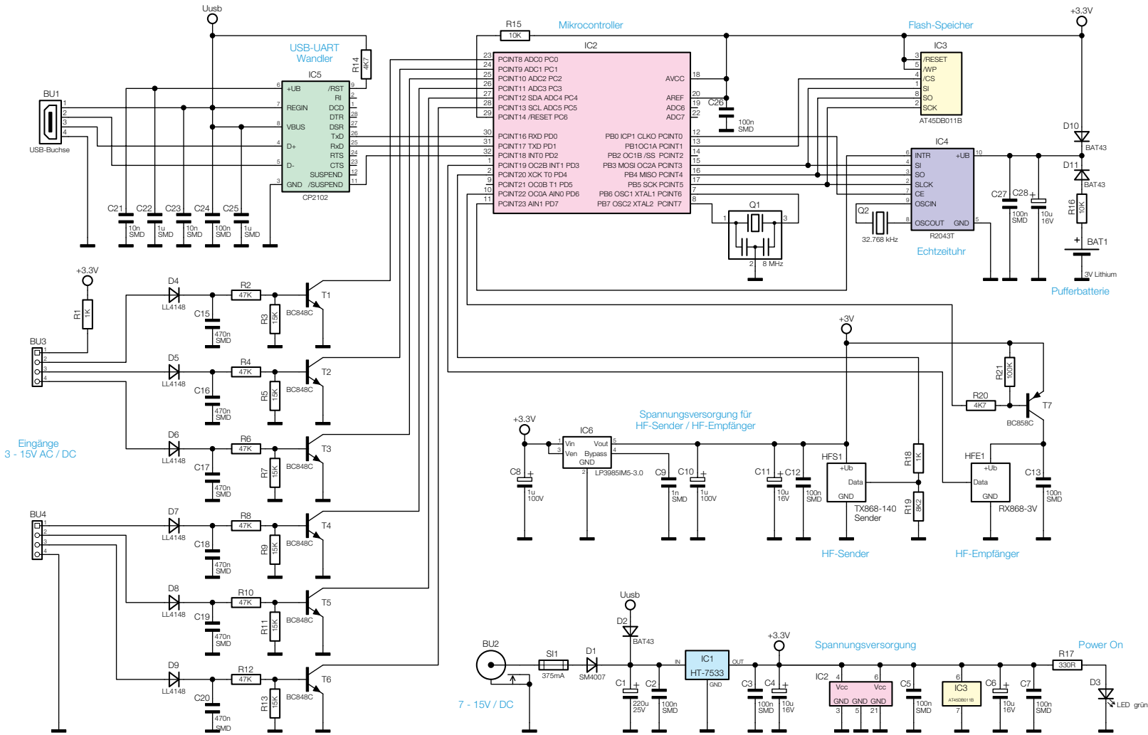
Bild 4: Schaltbild der Makrosteuerung FS20 MST 1
