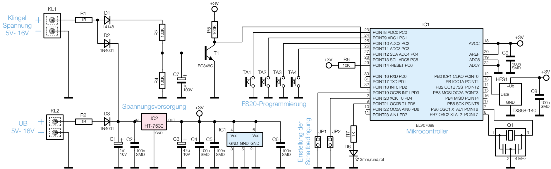
Bild 1: Schaltung der FS20-Klingelsignal-Erkennung
