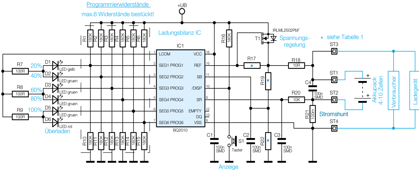
Bild 1: Schaltbild des NC/NiMH-Akku-Monitors
