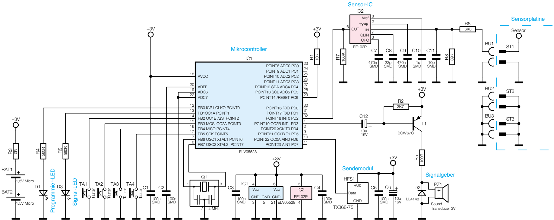
Bild 1: Schaltbild des Funk-Näherungsschalters FS20 SN
