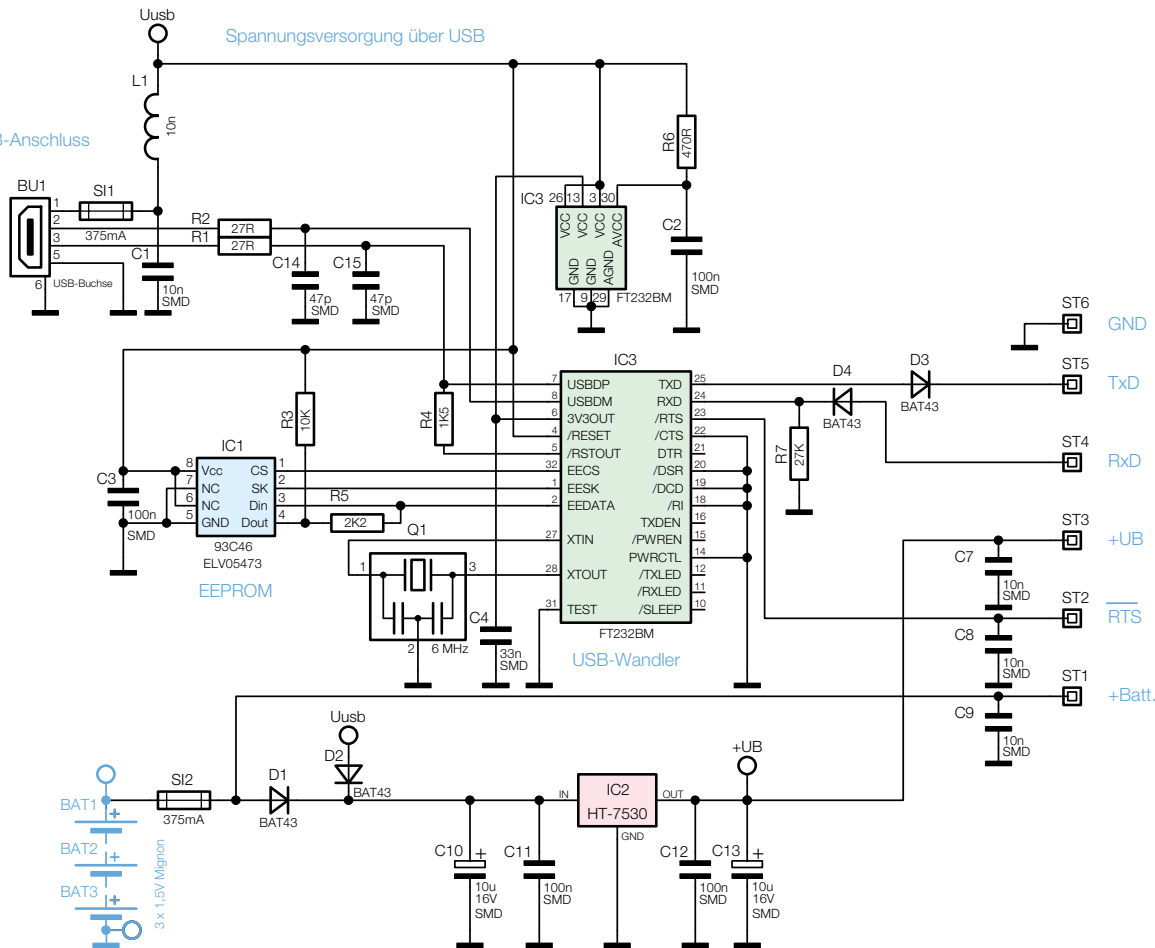
Bild 2: Schalt- bild der USB- Schnittstelle
